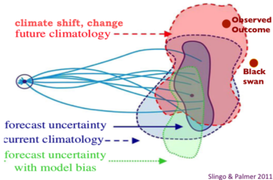
Abbildung 3: Ensembles und probabilistische Klimavorhersage
