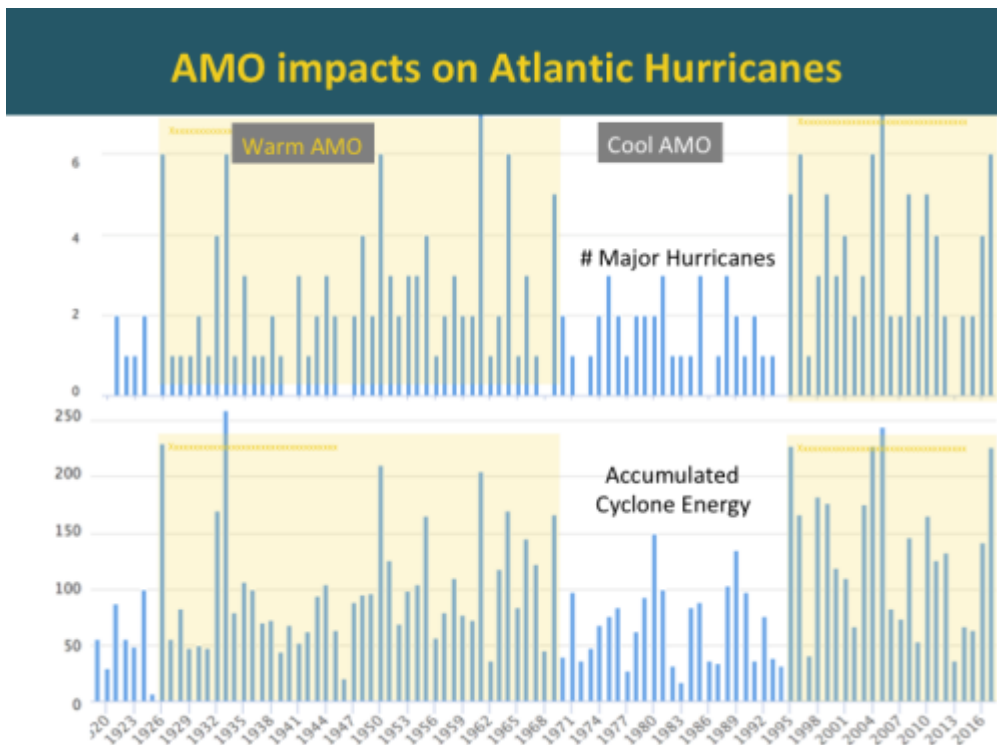
Abbildung 12: Auswirkungen der AMO auf atlantische Hurrikane
