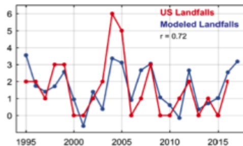
Abbildung 17: Vorhersage atlantischer Hurrikane: worst case -Szenario
