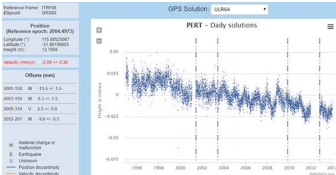
Abbildung 1 (oben) Fremantle, relativer mittlerer Meeresspiegel. Lineare und parabolische Fittings der PSMSL RLR Daten, wie sie vorhanden sind oder Lücken aufgefüllt. (unten) PERT (Perth) GPS-dome [Kuppel, ... ~Antenne – nicht mein Fachgebiet, aber offensichtlich handelt es sich um GPS gestützte Bojen, der Übersetzer]. Bild reproduziert und modifiziert von SONEL [Link unten erläutert]
