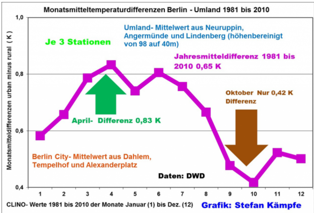
Grafik 5: In der CLINO- Normalperiode von 1981 bis 2010 gefundene UHI- Differenzen in Kelvin, gebildet aus den Mitteln dreier urbaner Stationen in Berlin und dreier ländlicher Stationen in Brandenburg. Hohen, verstädterungsbedingten Differenzen von über 0,8 K im April stehen geringere im Spätsommer/Frühherbst gegenüber. Die jahreszeitlich bedingten UHI- Effekte sind in Berlin eng mit geänderten Sonnenscheinverhältnissen und Großwetterlagenhäufigkeiten verknüpft.
