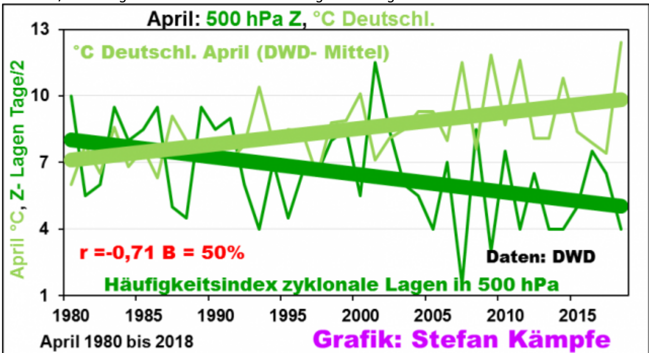
Grafik 7b: Seit 1980 liegen die Daten der Objektiven Wetterlagenklassifikation des DWD vor. Besonders stark kühlend wirken
