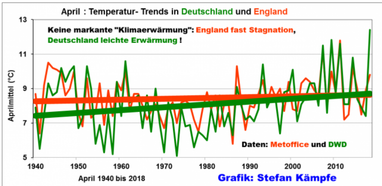
Grafik 11: Fast keine April- Erwärmung in England (orange) seit 1940. Der 2018er April blieb dort deutlich hinter den wärmsten Monaten der 1940er und der späten 1980er bis der frühen 2010er Jahre zurück.
