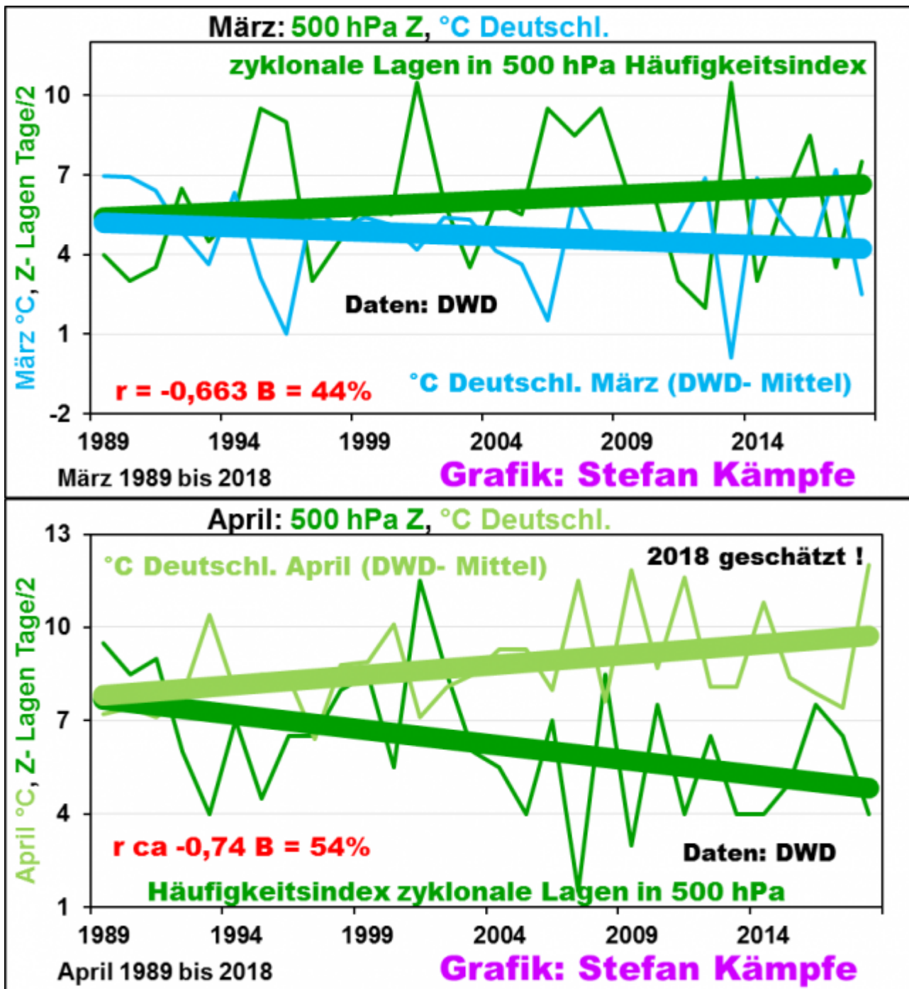
Abb. 8a und 8b: Leichte Märzabkühlung (8a, oben) seit 1989 auch wegen der leichten Häufigkeitszunahme der in der Höhe zyklonalen Großwetterlagen, welche auf höhenkalte Luft hinweisen. Zur Erwärmung hochreichender Kaltluft reicht die Kraft der Märzsonne nicht aus; besonders dann nicht, wenn Schnee liegt, so wie zeitweise auch im März 2018. Im April wirken dieselben Wetterlagen ebenfalls stark kühlend, aber da wurden sie seltener (8b, unten). Näheres zu Objektiven Wetterlagenklassifikation des DWD unter https://www.dwd.de/DE/leistungen/wetterlagenklassifikation/beschreibung.html?nn=16102&lsbId=375412
