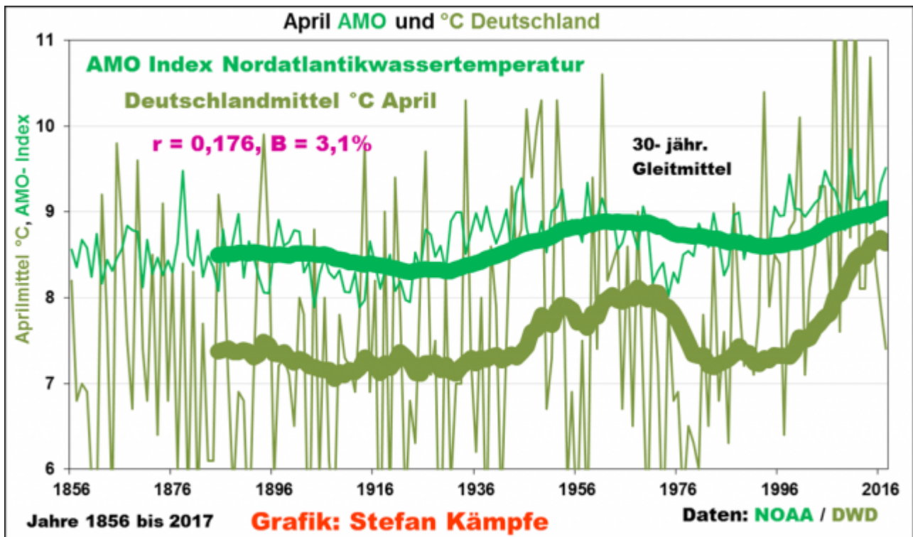
Abb. 12: Die AMO (Atlantische Mehrzehnjährige Oszillation, ein Maß für die Schwankung der Wassertemperatur im zentralen Nordatlantik) weist in der Mitte des 20. Jahrhunderts und gegenwärtig Warmphasen auf, in welchen tendenziell auch der April in Deutschland milder ausfiel.
