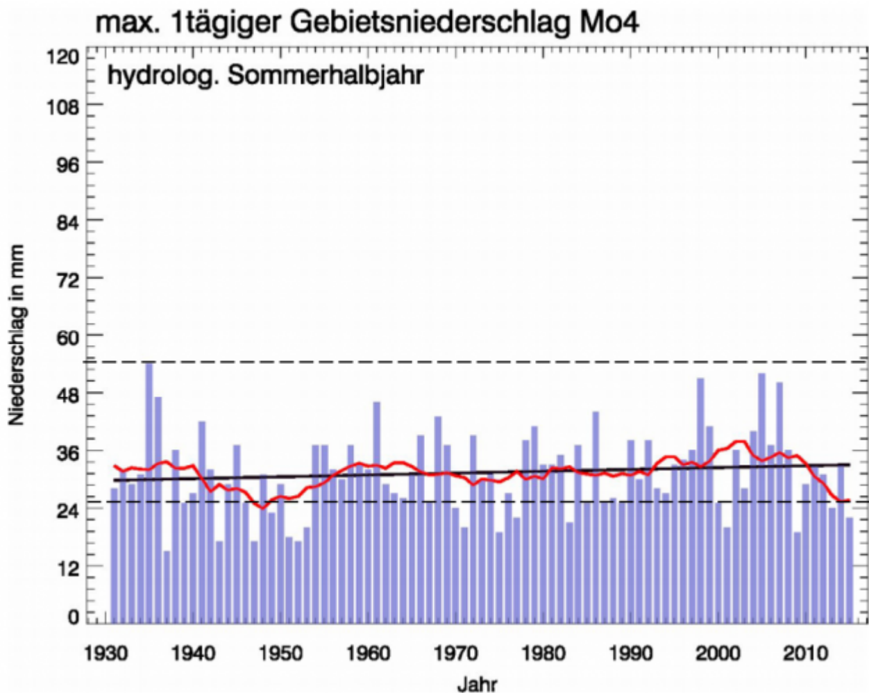
Bild 6.2 [1] Gebiet Mo4, Verlauf Starkregenereignisse Sommerhalbjahr von 1931 – 2015. Hilfslinien vom Autor ergänzt
