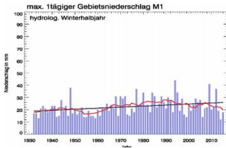
Bild 11 [1] Gebiet M1 (+31,4 % Winterhalbjahr). Verlauf Winterhalbjahr, Sommerhalbjahr Starkregenereignisse
