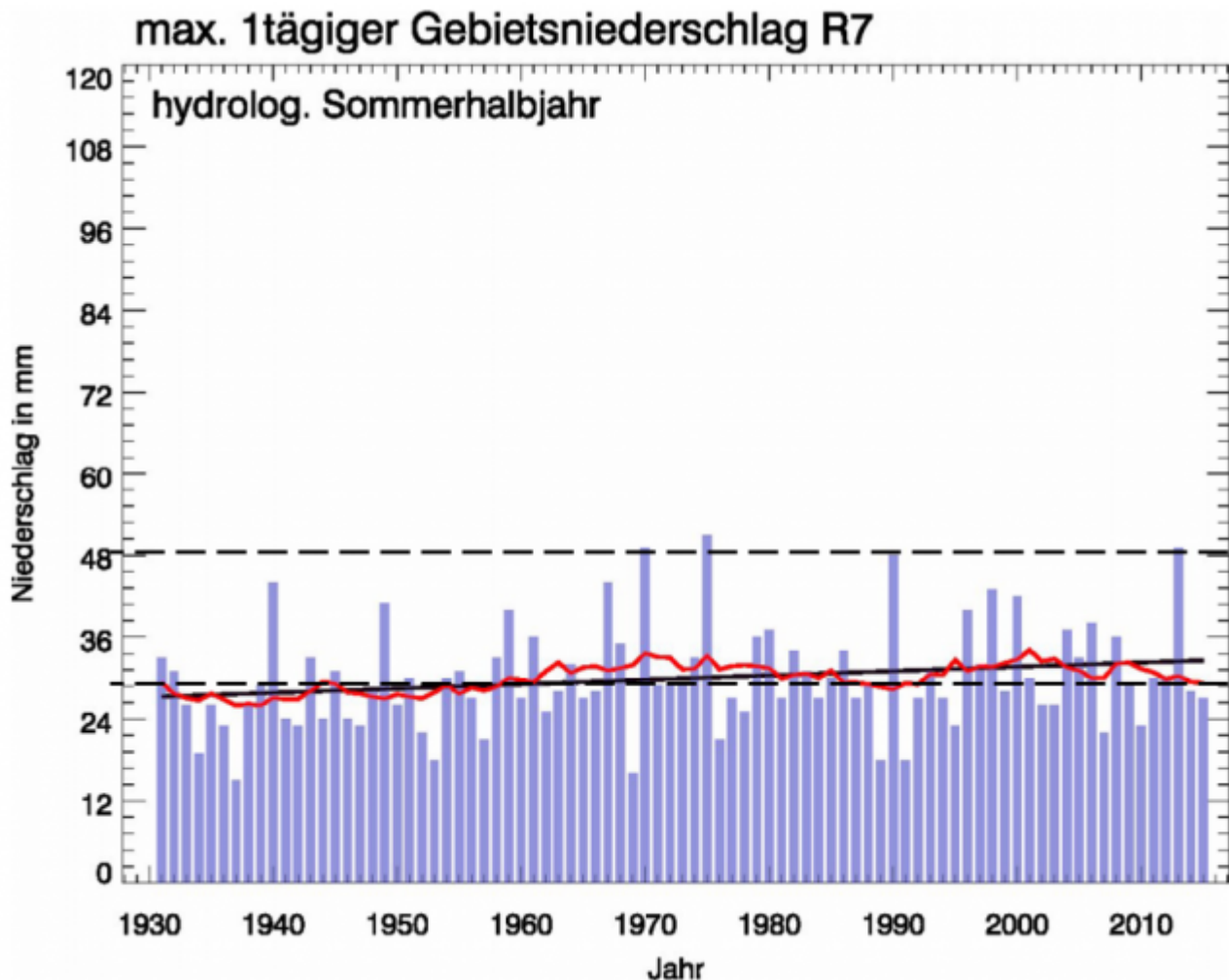
Bild 6.1 [1] Gebiet R7, Verlauf Starkregenereignisse Sommerhalbjahr von 1931 – 2015. Hilfslinien vom Autor ergänzt
