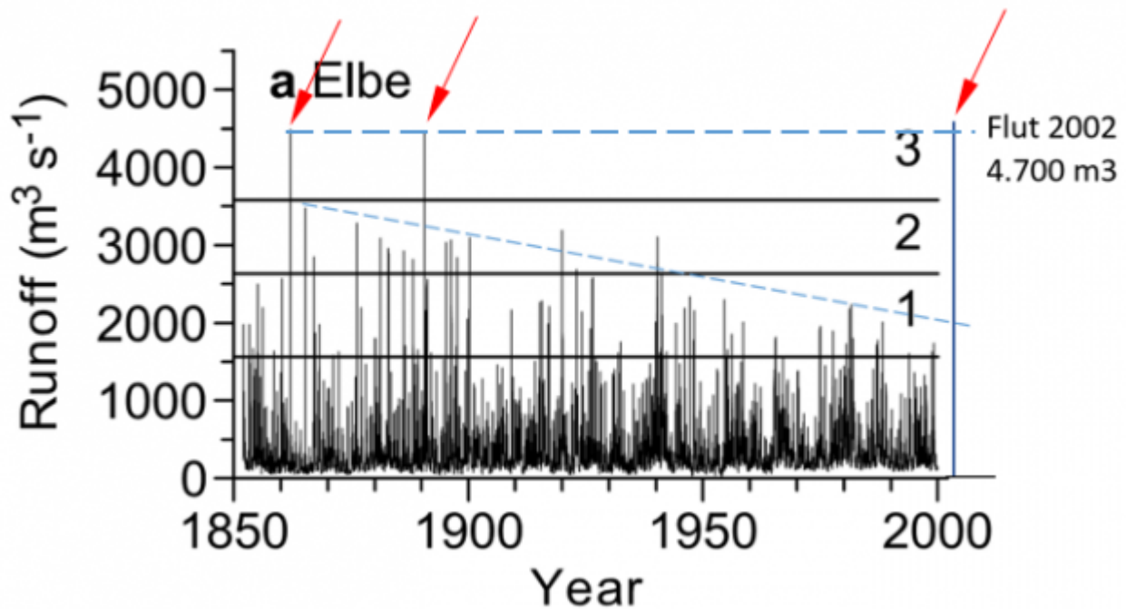
Bild 19.2 Elbe, Fließmengen seit 1850. Wert der Flut 2002 von 4.700 m 3 nach vom Autor nach den Angaben in der Studie ergänzt. Quelle: MUDELSEE ET AL.: EXTREME FLOODS IN CENTRAL EUROPE
