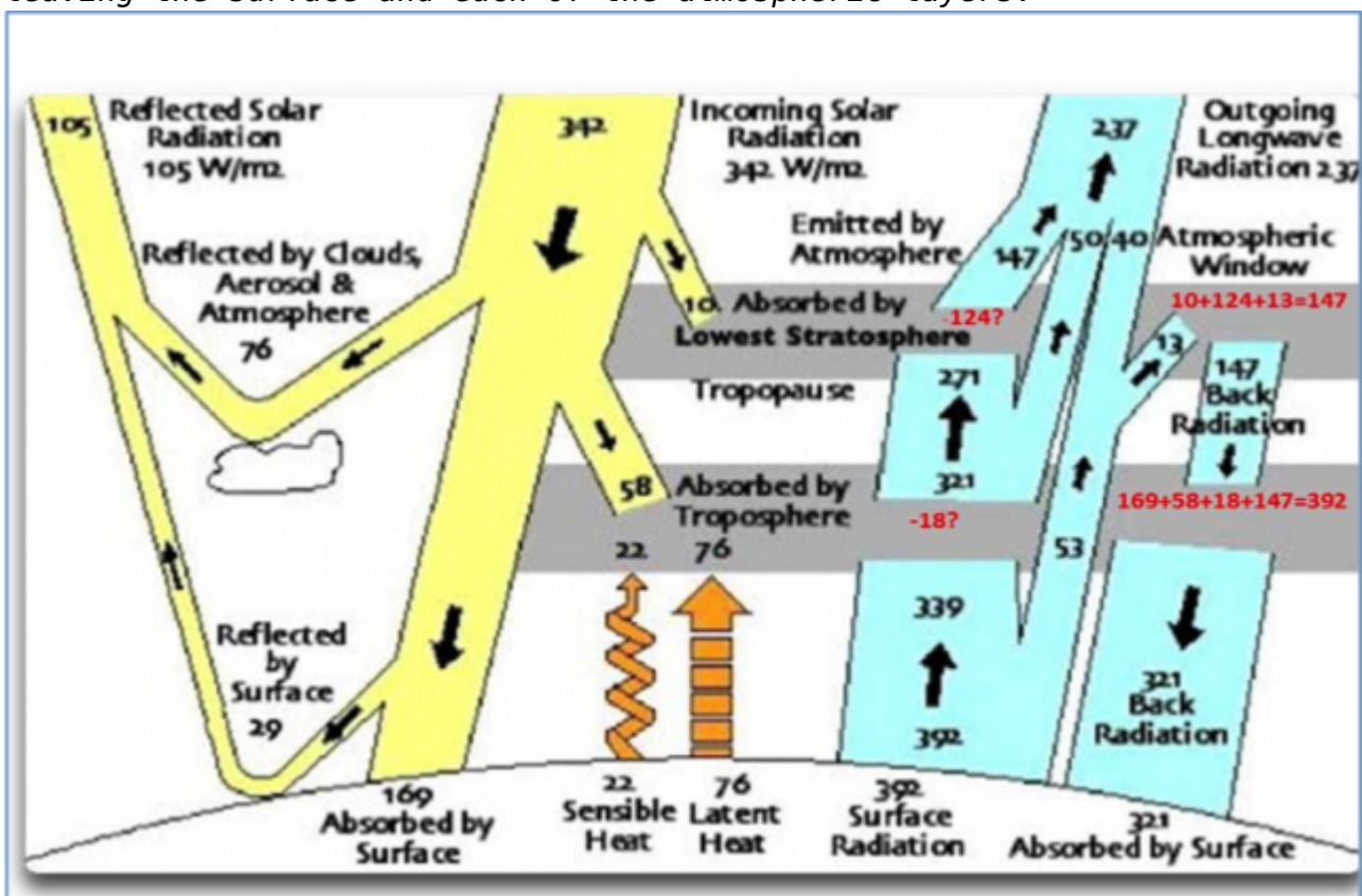
Abbildung 2: Globales Energiebudget nach Kiehl&Trenberth aus Eschenbach @ WUWT
