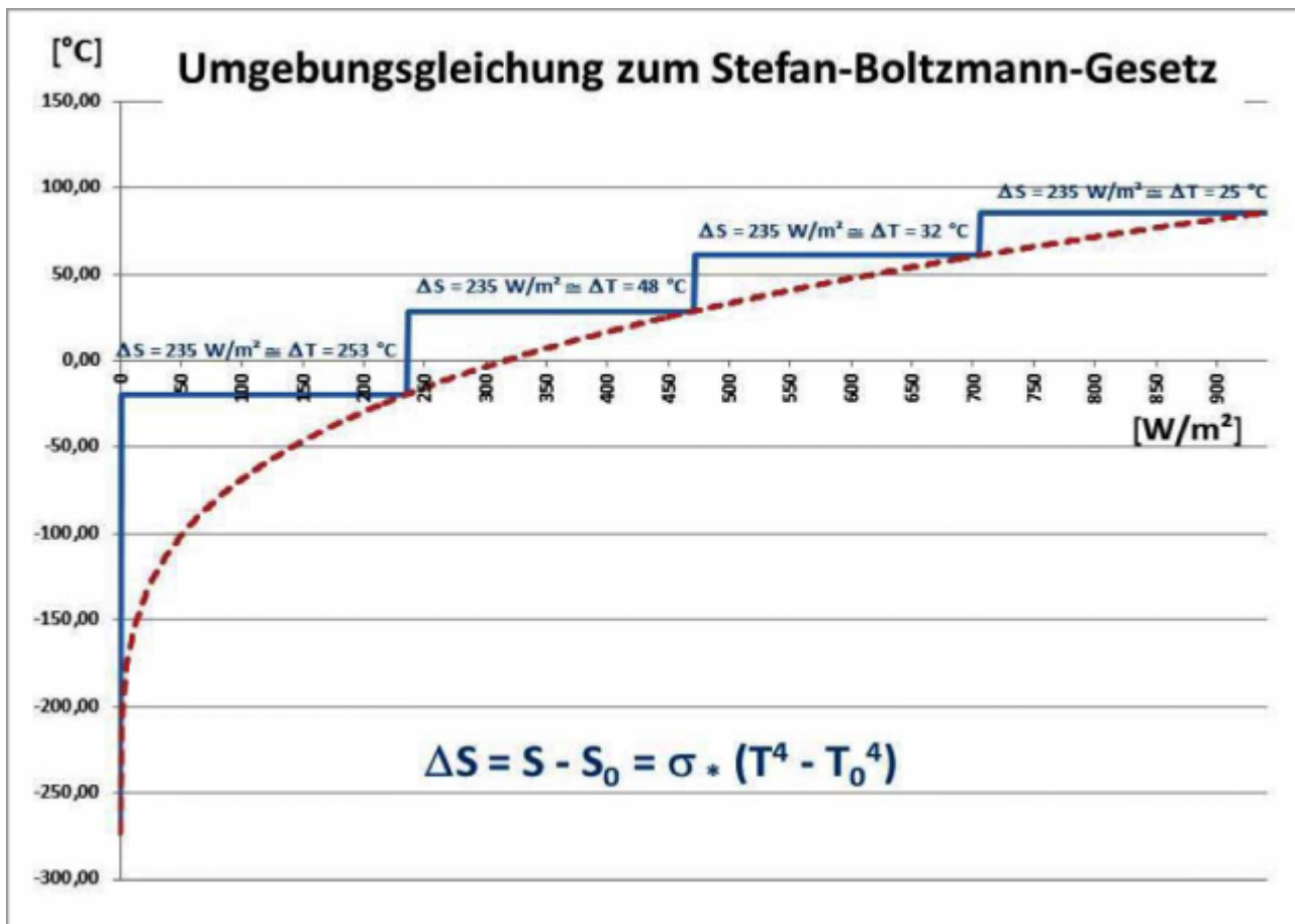
Abbildung 4: Die Umgebungsgleichung des Stefan-Boltzmann-Gesetzes Rot gestrichelt: Die T^4 -Beziehung des S-B Gesetzes zwischen Strahlung und Temperatur
