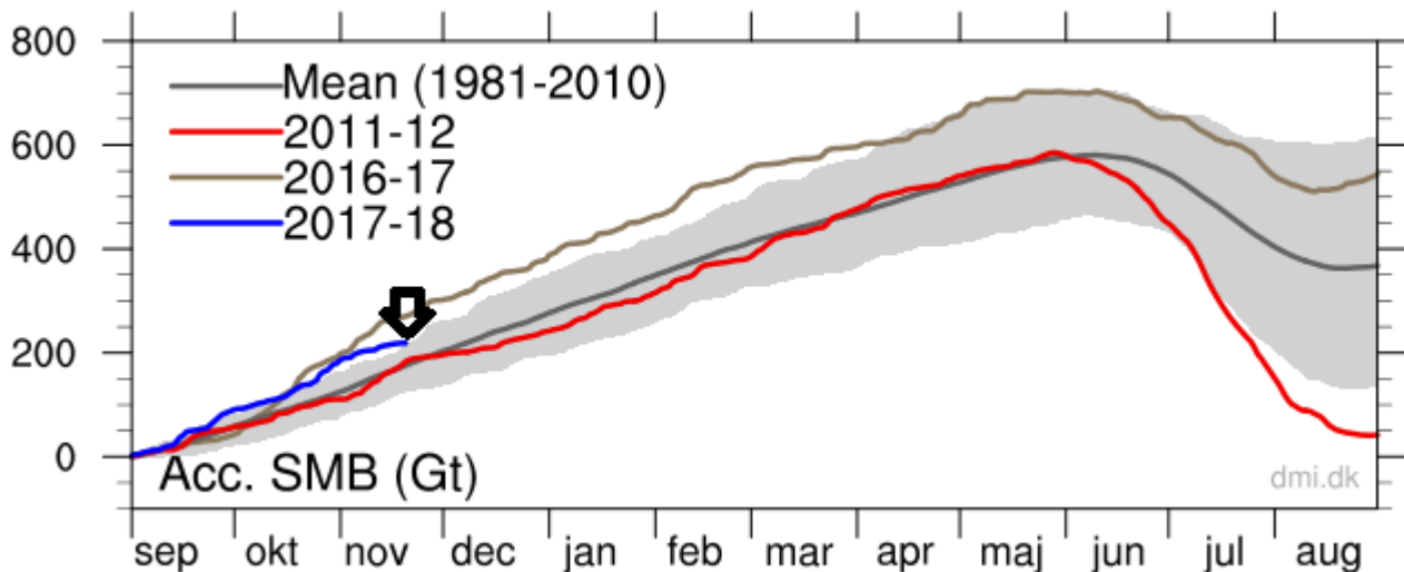
Abbildung: Akkumulierte Oberflächen-Massenbilanz vom 1. September bis heute (blaue Linie, Gt) im Vergleich zur Massenzbilanz der Saison 2011-12 (rot). Damals war es zu einem sehr hohen sommerlichen Abschmelzen in Grönland gekommen. Zum Vergleich ist die Mittelkurve der Jahre 1981 bis 2010 eingezeichnet (grau). Quelle: Danish Meteorological Institute.
