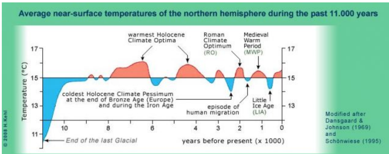
Abb. 1: Nordhemisphärische Temperaturen seit der letzten Eiszeit
