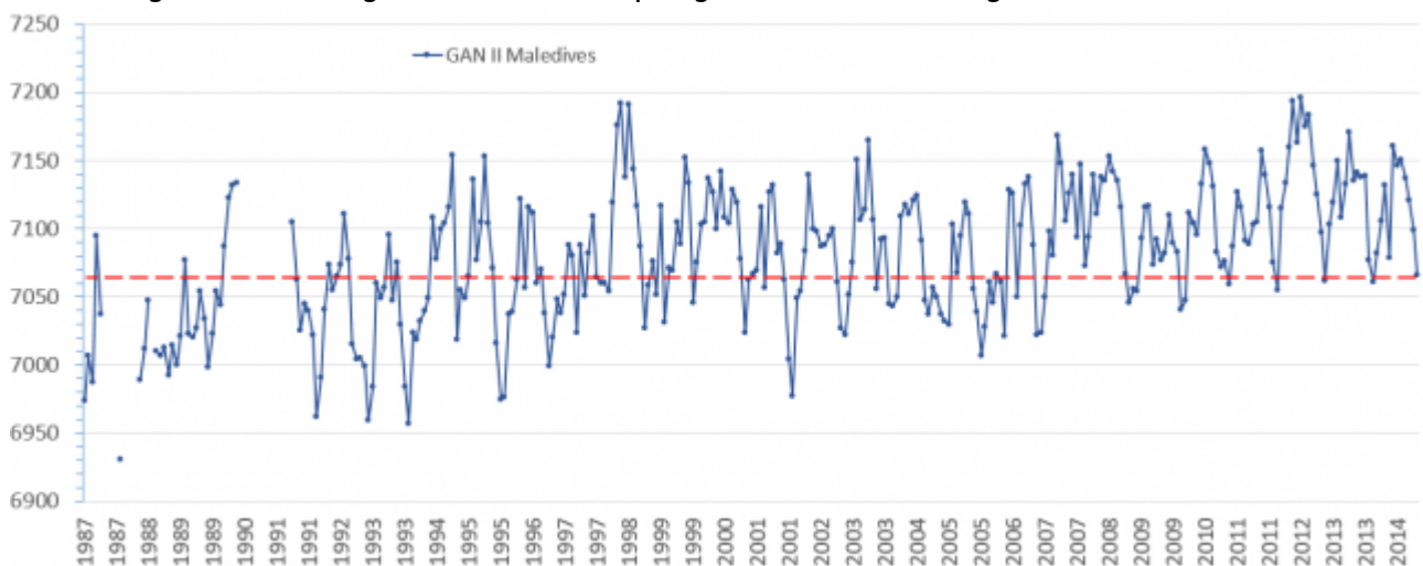
Bild 3 Verlauf des Seepiegels bei den Malediven 1983 – 2014. Bild vom
