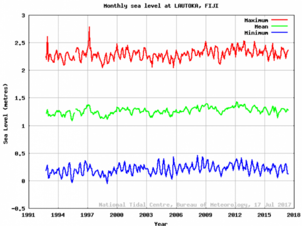
Bild 11 Pegelverlauf Fidji von Ca. 1993 – Juli 2017
