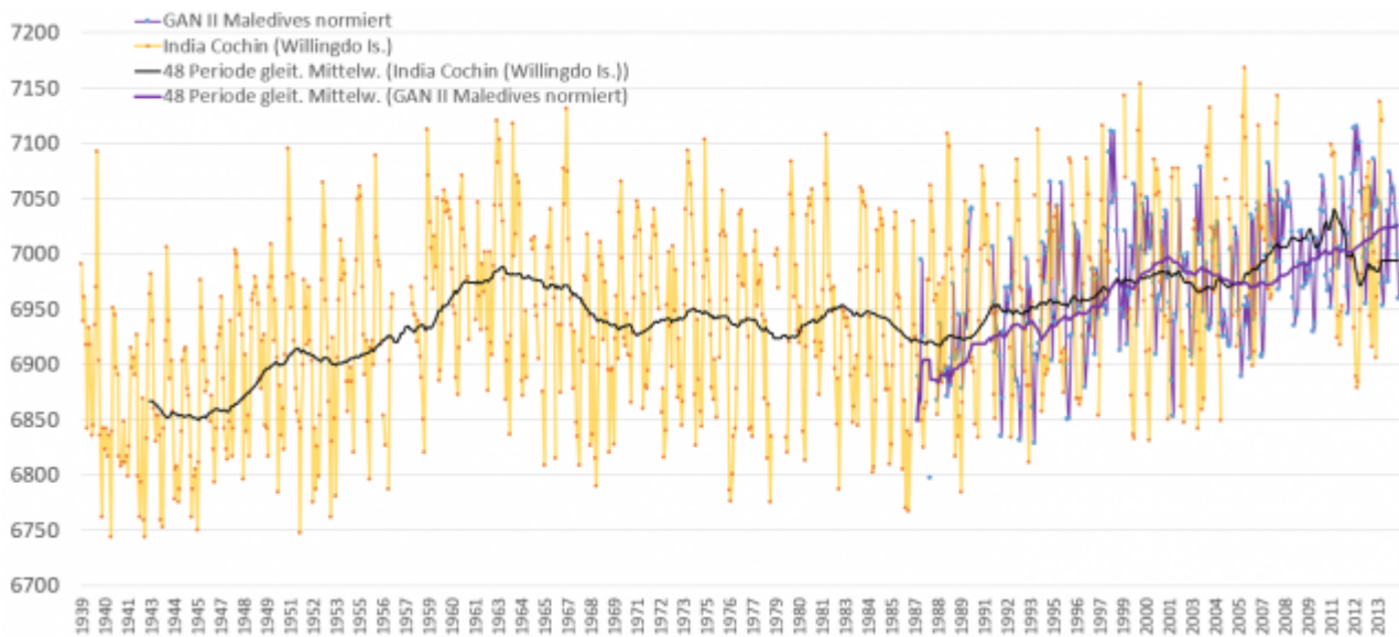
Bild 4 Verlauf Seepegel Malediven und gegenüber liegendes Festland von Indien. Daten Maledives gedehnt und im Offset angepasst. Grafik vom Autor anhand der PSMSL-Daten erstellt
