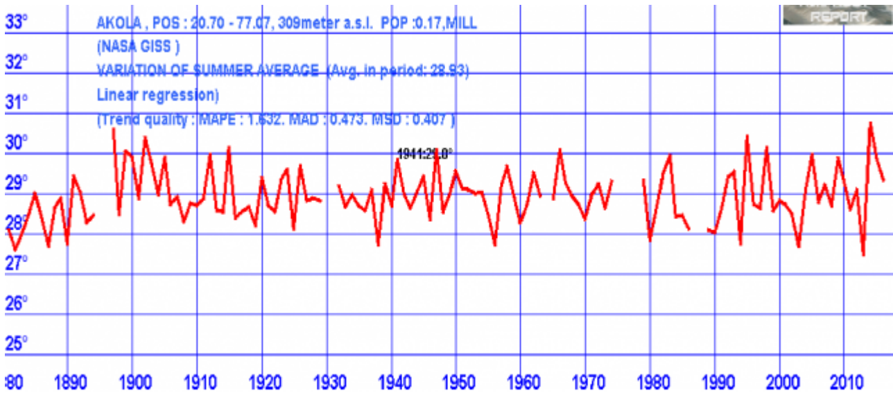
Bild 10 Sommertemperatur Indien, Akola von 1880 ... 2015. Quelle: RIMFROST Viewer
