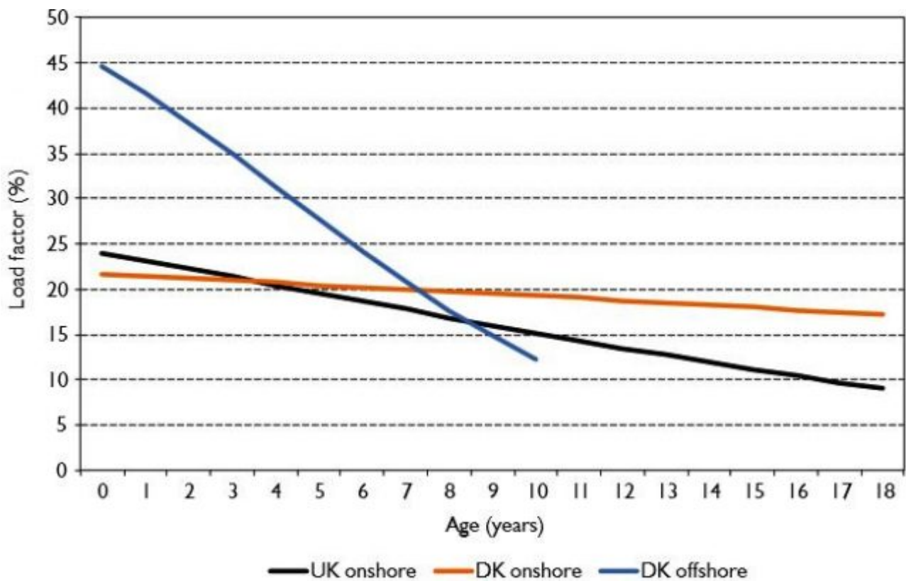
Abb. 14: Windkraftanlagen an Land (schwarz: Großbritannien, orange Dänemark) „starten“ ihren Regelbetrieb mit durchschnittlich nur etwa 20 bis 25% ihrer Nennleistung und büßen pro Jahr 1 bis 2% dieser Leistung ein; nach 18 Jahren sind es noch 9 bis 17%. Offshore-Anlagen (blau) starten zwar mit verlockenden 45% der Nennleistung, büßen aber pro Jahr etwa 6% ein und sind daher bereits nach 10 Jahren Regelbetrieb auf etwa 12% ihrer Nennleistung abgestürzt. Bildquelle (11)
