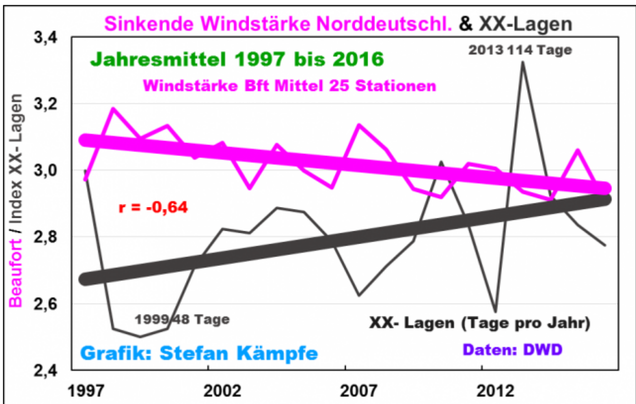
Abb. 5: Im Mittel der 25 Stationen aus Norddeutschland sank die Windgeschwindigkeit um 0,15 Beaufort. In dem Datensatz ist auch der Brocken, Norddeutschlands einziger hoher Berg, enthalten, an dem der Wind gleichfalls schwächer wurde, was nahelegt, dass geänderte Luftdruckverhältnisse zumindest mitverantwortlich für die Windabnahme waren (die zumeist windschwachen XX- Lagen, solche ohne eindeutige Anströmrichtung, sind tendenziell häufiger geworden, und ihre Häufigkeit korreliert recht gut mit der Windgeschwindigkeit).
