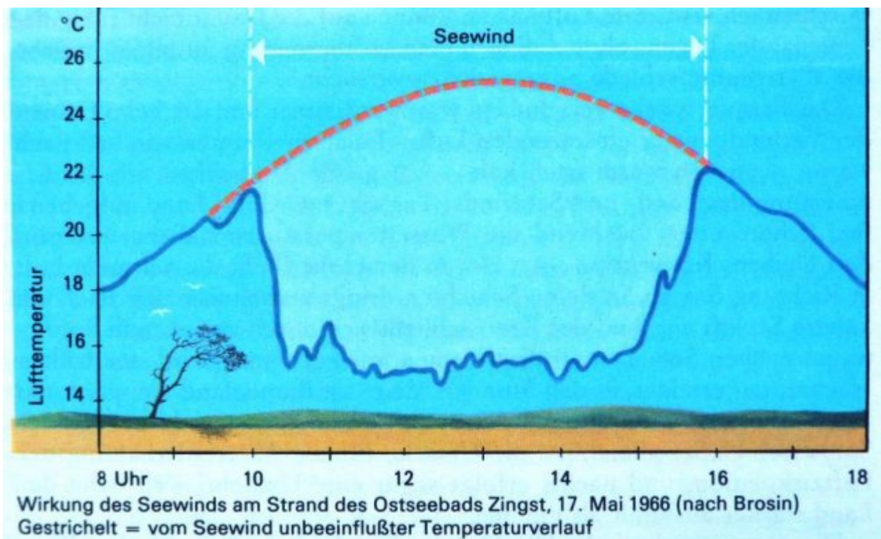
Abb. 11: In der Grafik ist nicht die Windstärke, sondern der Gang der Lufttemperatur an der Ostseeküste an einem sonnigen, von Hochdruckwetter beeinflussten Tag gezeigt. Nur während der Seewind-Phase, die in diesem Beispiel von etwa 10 bis 16 Uhr Normalzeit dauerte, steht ausreichend Wind zur Stromerzeugung zur Verfügung. Der Seewind gibt sich durch seine Kühlungswirkung zu erkennen; er verursachte am Vormittag einen Temperatursturz von etwa 6 Grad. Bildquelle (8)
