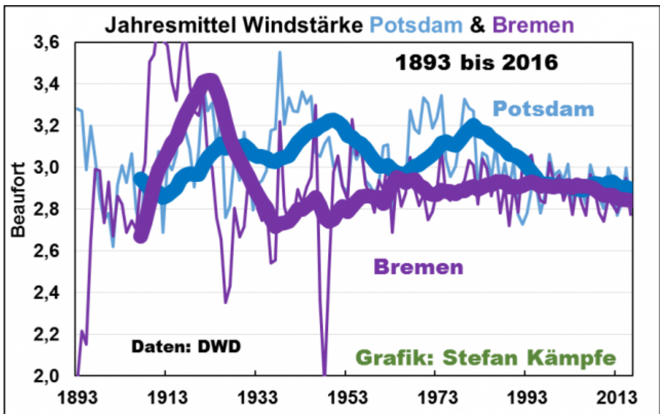
Abb. 3: An beiden Stationen schwankte die Windstärke (Jahresmittel) erheblich. An der Nordsee scheint um 1915 besonders viel und in den 1930er bis 1950er Jahren eher wenig Wind geweht zu haben, in Potsdam waren die 1930er bis 1940er sowie die 1970er Jahre windig (das endbetonte Gleitmittel „hinkt“ nach). Erst seit den 1990er Jahren verhalten sich beide Reihen ähnlich.
