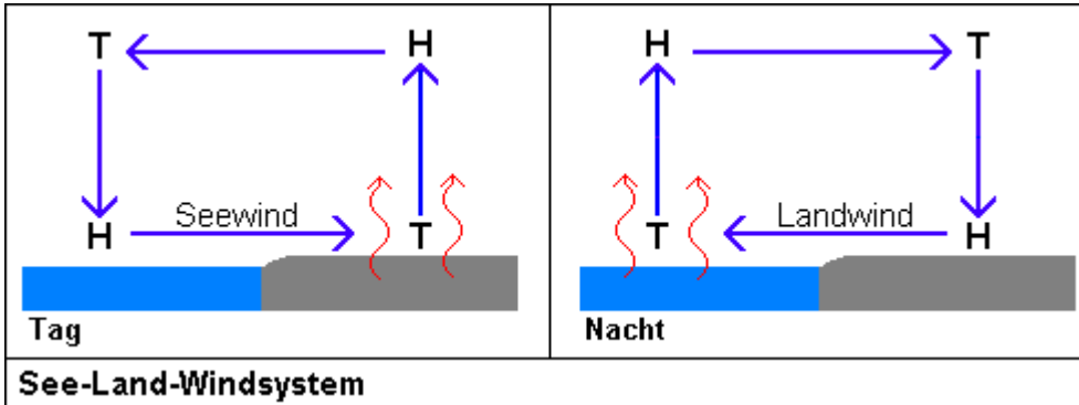
Abb. 10: Land-/Seewindsystem (Quelle: Google). Im Sommer ist es besonders ausgeprägt.
