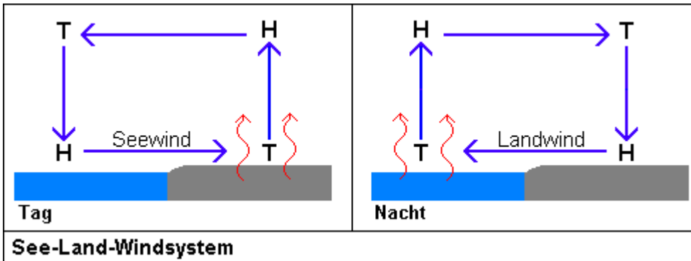
Abb. 10: Land-/Seewindsystem (Quelle: Google). Im Sommer ist es besonders ausgeprägt.
