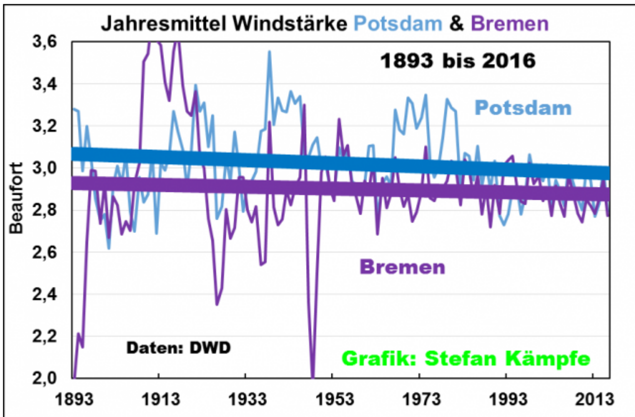
Abb. 4: Seit 1893 nahm die Windgeschwindigkeit leicht ab; in Potsdam etwas stärker als in Bremen.
