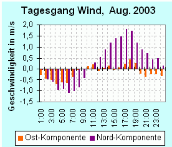
Abb. 7: Tagesgang der Windstärke in Jena (Abweichungen vom Mittelwert) im von Hochdruckwetter dominierten August 2003. Man erkennt ein Minimum am frühen Morgen- wenn im einsetzenden Berufsverkehr besonders viel Strom verbraucht wird. Bildquelle (7)
