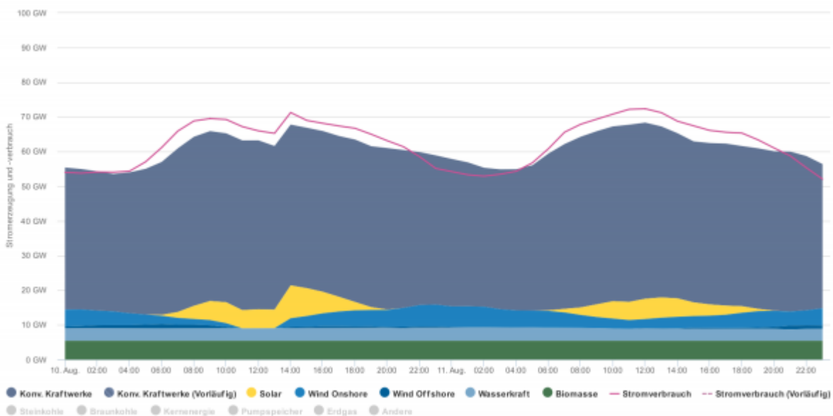
Abb. 9: Wenig Sommersonne und wenig Wind – fast eine sommerliche „Dunkelflaute“ am 10./11.08. 2017. Wieder musste fast aller Strom konventionell erzeugt werden. Trotz aller vollmundigen Versprechen steckt die „Energiewende“ in einer tiefen Krise. (Bildquelle: Agora Energiewende)
