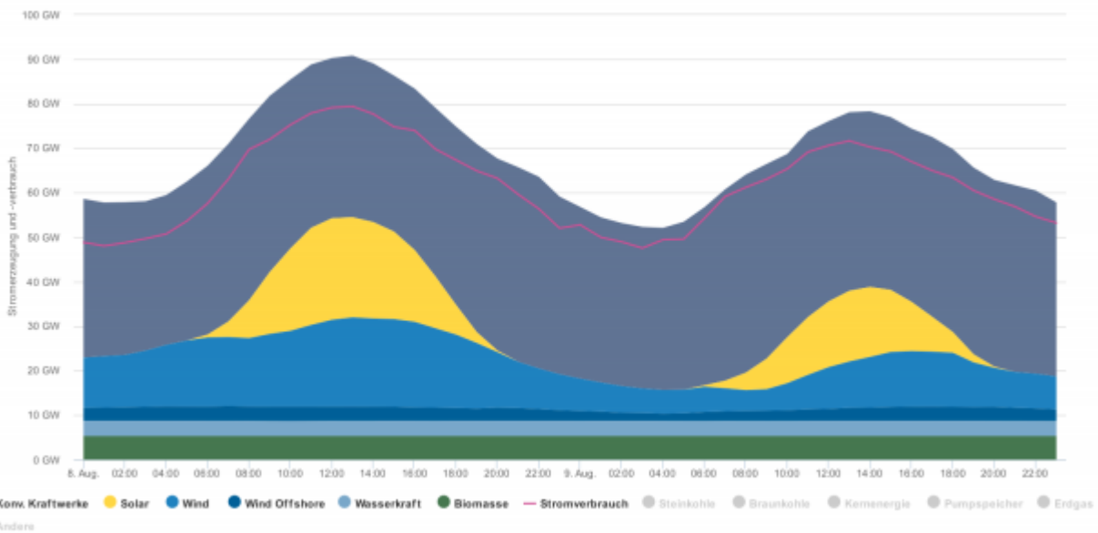
Abb. 8: Sehr viel Sonne und mehr Wind gegen Mittag am 08. und 09.08.2016 („Mittags-Schwemme“). Aber selbst da mussten noch erhebliche Strommengen konventionell erzeugt werden, besonders in den Nächten war deren Anteil sehr hoch. (Bildquelle: Agora Energiewende)
