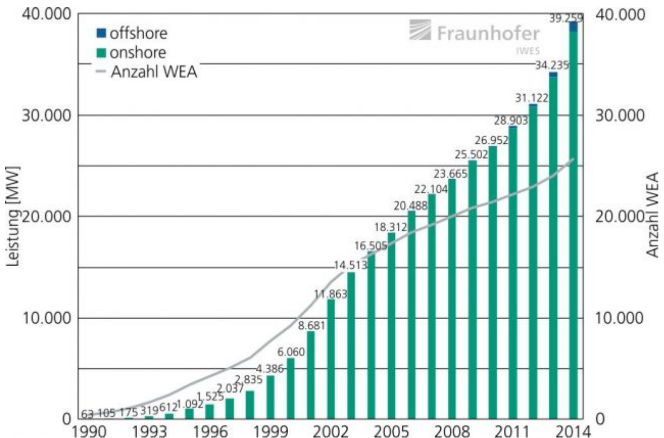
Abb. 1: In Deutschland begann der massive Windkraft- Ausbau nach der Mitte der 1990er Jahre. Er setzte sich auch nach 2014, dem Endpunkt dieser Grafik, weiter fort. Bildquelle (2)
