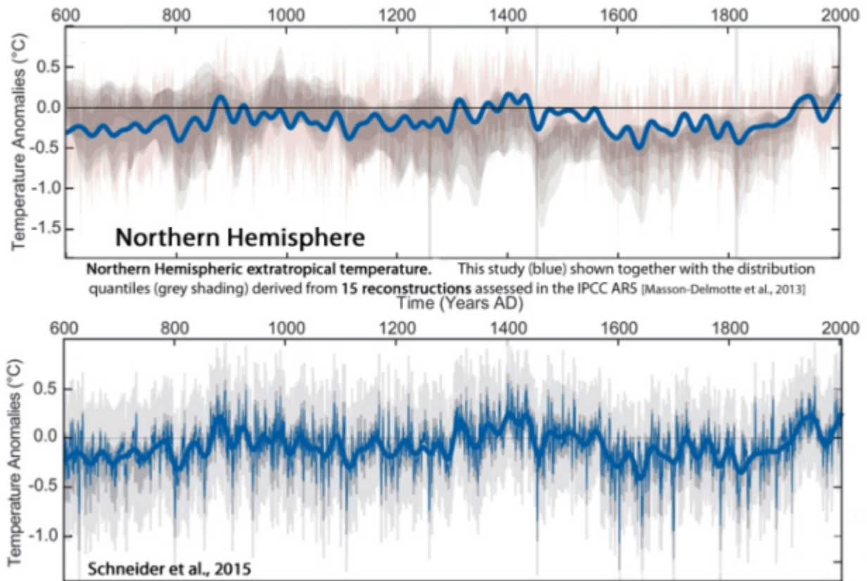
Bild 1-19 [30] Proxi-Temperaturrekonstruktion Nordhemisphere
