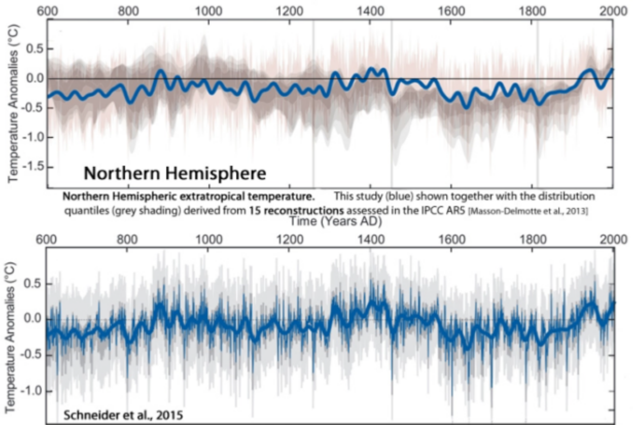
Bild 1-19 [30] Proxi-Temperaturrekonstruktion Nordhemisphere
