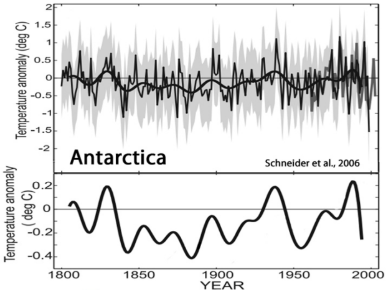
Bild 1-20 [30] Proxi-Temperaturrekonstruktion Antarktis
