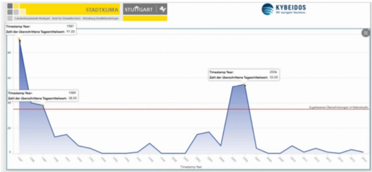
Abb.38, Quelle: ( https://www.youtube.com/watch?v=tSjEWBD6WmA ), „Beispielszenario Feinstaubanalyse“ zeigt die Feinstaubdatenreihe (Zahl der überschrittenen Tageshöchstwerte) Stuttgart-Mitte von 1987 bis 2016. Deutlich hat sich die Luftqualität in Stuttgart verbessert. Die Zahl der sog. Feinstaubalarmlage ist verschwindend gering. Kein Anlass für irgendwelche Maßnahmen, wie Fahrverbote.
