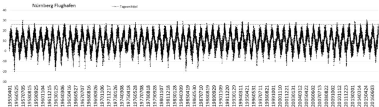
Bild 3 Nürnberg Tageswerte 1950 – 31.06.2017. Quelle: DWD
