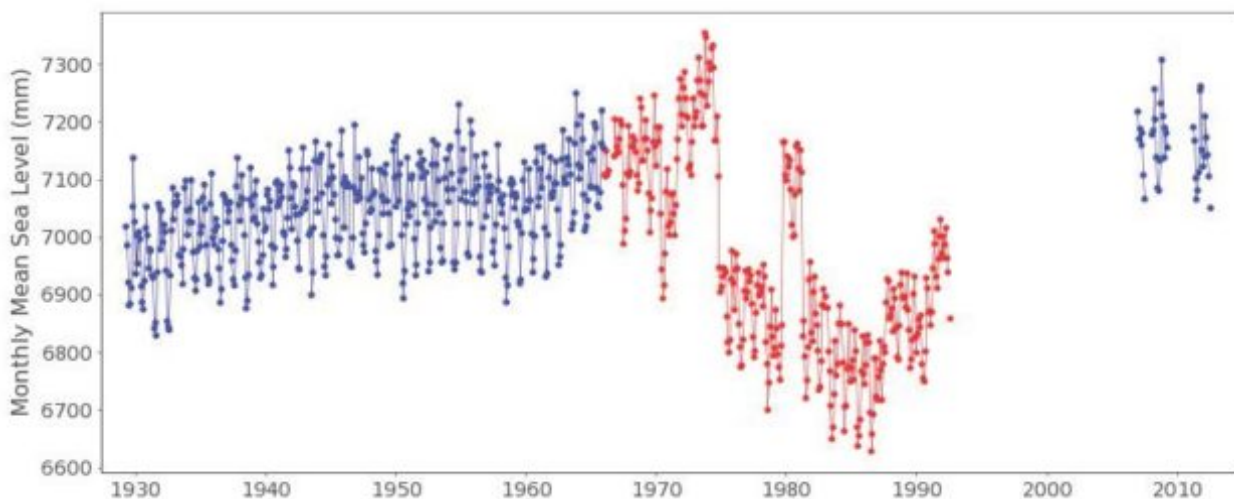
Bild 1: Monats-Meeresspiegel-Höhen von Takoradi [mm] (über dem
