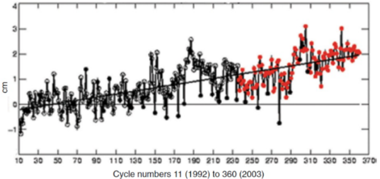
Bild 3 [3] Satelliten-Pegolverlauf nach der Adjustierung
