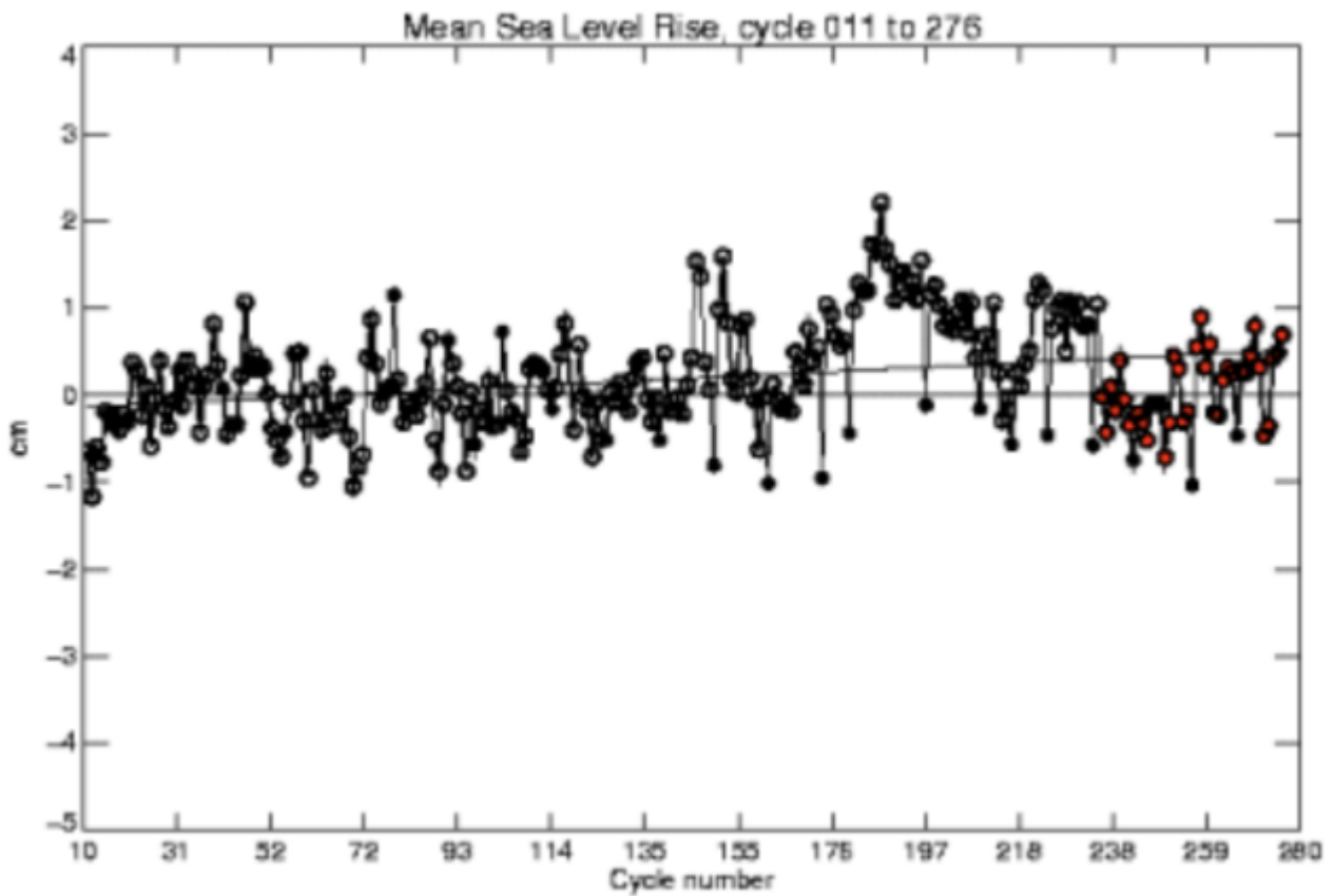
Bild 2 [3] Satelliten-Pegolverlauf vor der Adjustierung
