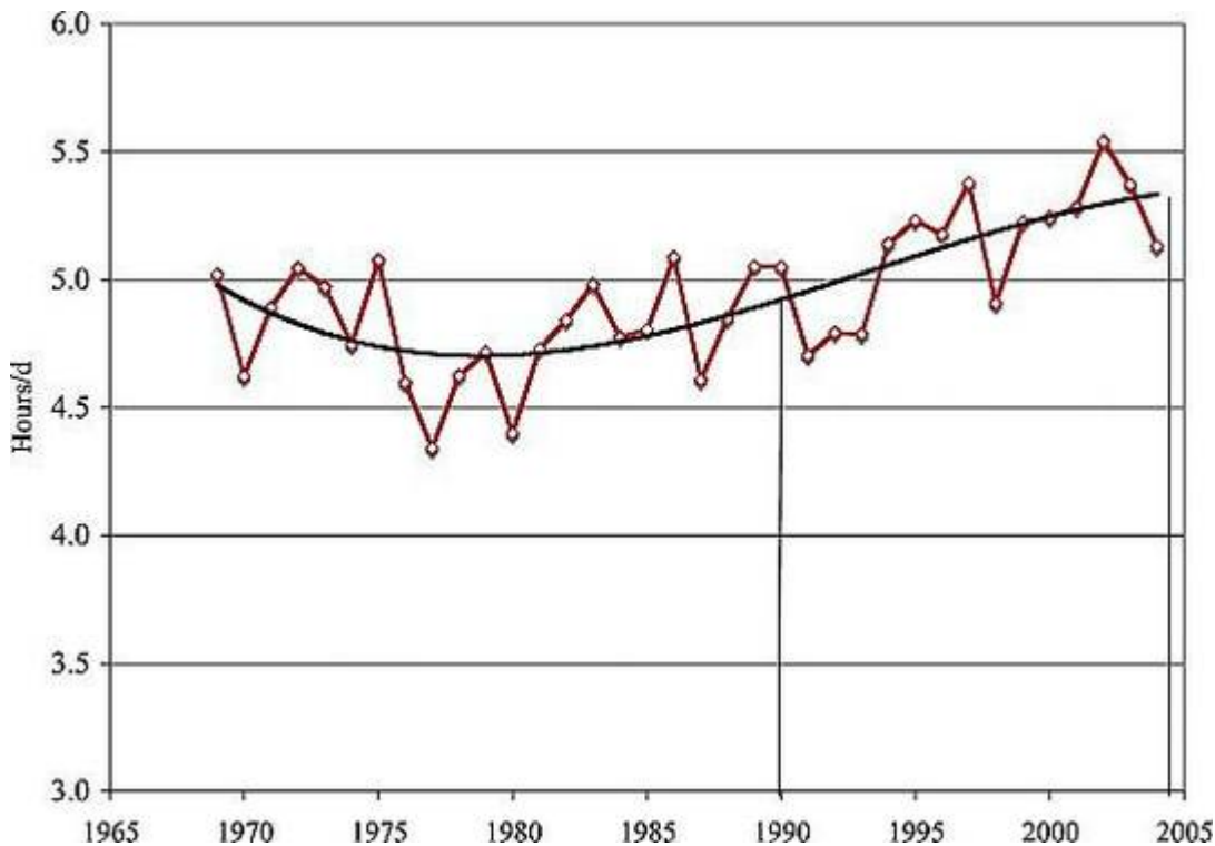
Abbildung 7: Mittel der täglichen Sonnenscheindauer (Stunden) pro Jahr mit Beobachtungswerten aus Odessa, Moskau, Tartu (Estland), der Schweiz und Tateno/Japan. (Quelle http://onlinelibrary.wiley.com/doi/10.1029/2008JD011290/full#footer-citing ).
