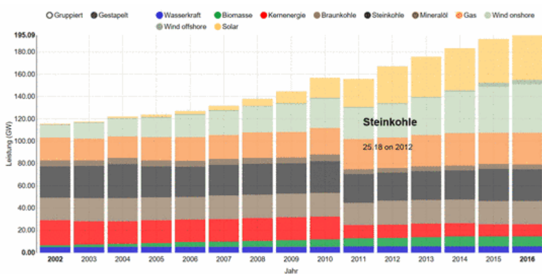
Bild 10 Installierte Nettoleistungen Deutschland gestapelt dargestellt. Quelle: Fraunhofer ISE Energy Charts
