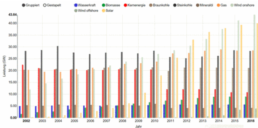
Bild 9 Installierte Nettoleistungen Deutschland gruppiert dargestellt. Quelle: Fraunhofer ISE Energy Charts
