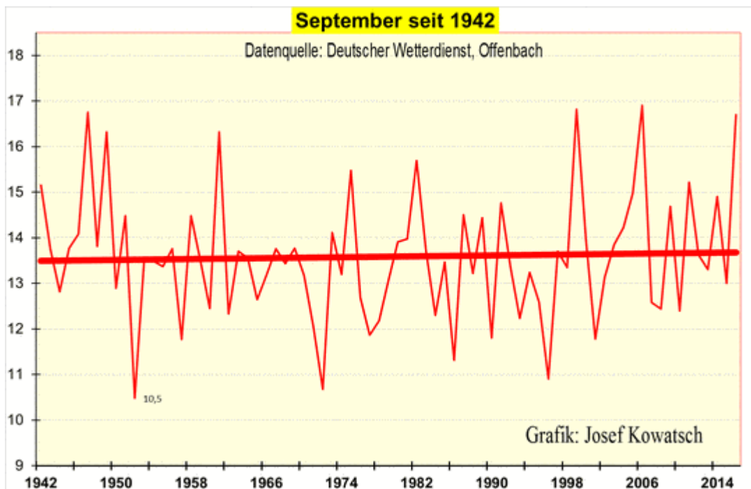
Abb.1: September 1942 bis 2016: Das sind 75 Jahre, weil 75 Septembermonate. Die Grafik zeigt, dass der September 2016 zu den wärmeren gehört. Die Trendlinie zeigt aber auch, dass in den letzten 75
