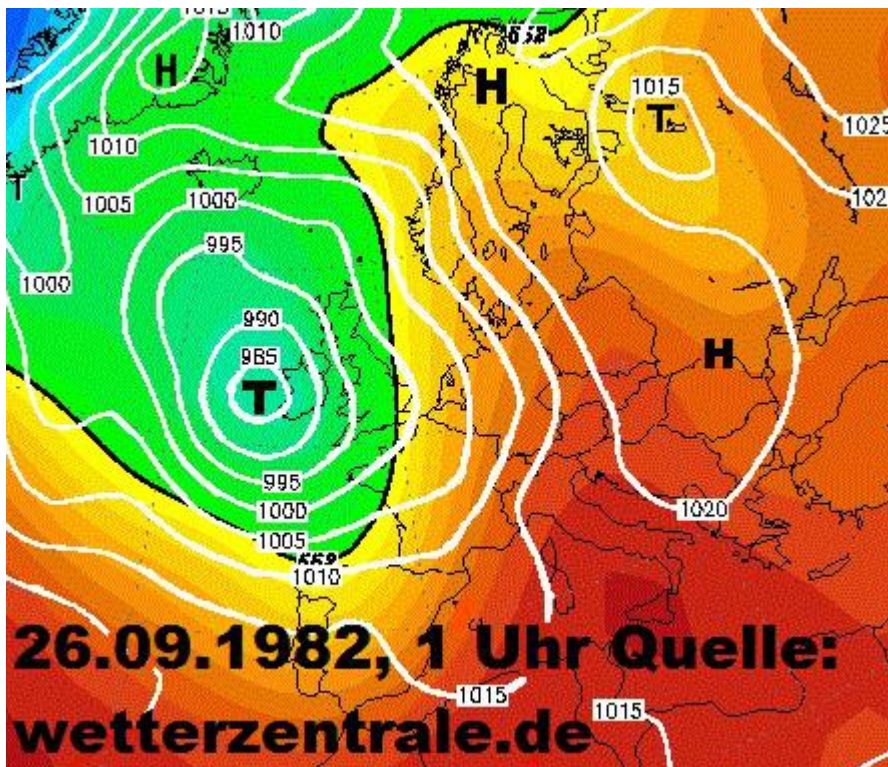
Abb. 7: Am 26.09.1982 herrschte eine der Situation von Mitte September 2016 vergleichbare Situation. Man erkennt wieder die Hochdruckzone Skandinavien/Balkan und ein kräftiges Tief, diesmal westlich von Irland. Über Deutschland wehte eine Südwind.
