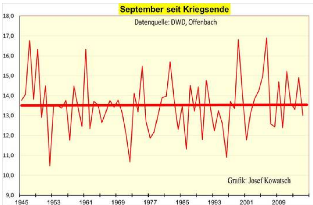
Abb. 2: Keine Septembererwärmung in Deutschland seit über 70 Jahren. In diesem Zeitraum nahm die CO 2 - Konzentration in der Atmosphäre um etwa 90ppm zu; das entspricht einer Steigerung um etwa 30%. Man achte auf die sehr warmen September 1947, 1949 und 1961. Erst 1999 und 2006 wurden deren Werte wieder erreicht beziehungsweise knapp übertroffen.
