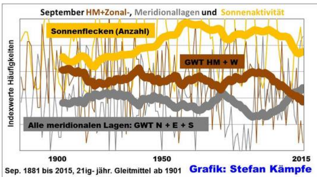
Abb. 8: Man achte besonders auf das spiegelbildliche Verhalten der jährlichen Sonnenaktivität (obere, gelbe Kurve) und der Häufigkeit der zu Extremwetter neigenden „meridianen“ oder „meridionalen“ Lagen im September (untere, graue Kurve). Die für den September eigentlich typischen, gemäßigten West- und Zentralhochlagen werden neuerdings hingegen seltener; ob sich dieser Trend fortsetzt, bleibt abzuwarten. Hinweis: Die Sonnenfleckenanzahl bildet die eigentliche Sonnenaktivität (Magnetismus, UV- und Röntgenstrahlung, Radiostrahlung und „Sonnenwind“) nur grob ab; sie ist jedoch als einzige Größe über lange Beobachtungszeiträume sicher verfügbar.
