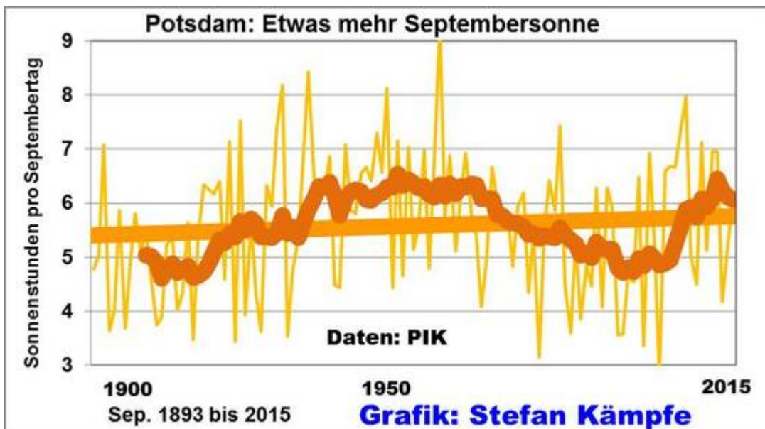
Abb. 4: Leicht zunehmende Sonnenscheindauer im September in Potsdam. Für ganz Deutschland fehlen leider langfristige Aufzeichnungen, doch dürfte auch im ganzen Land der September etwas sonniger geworden sein.
