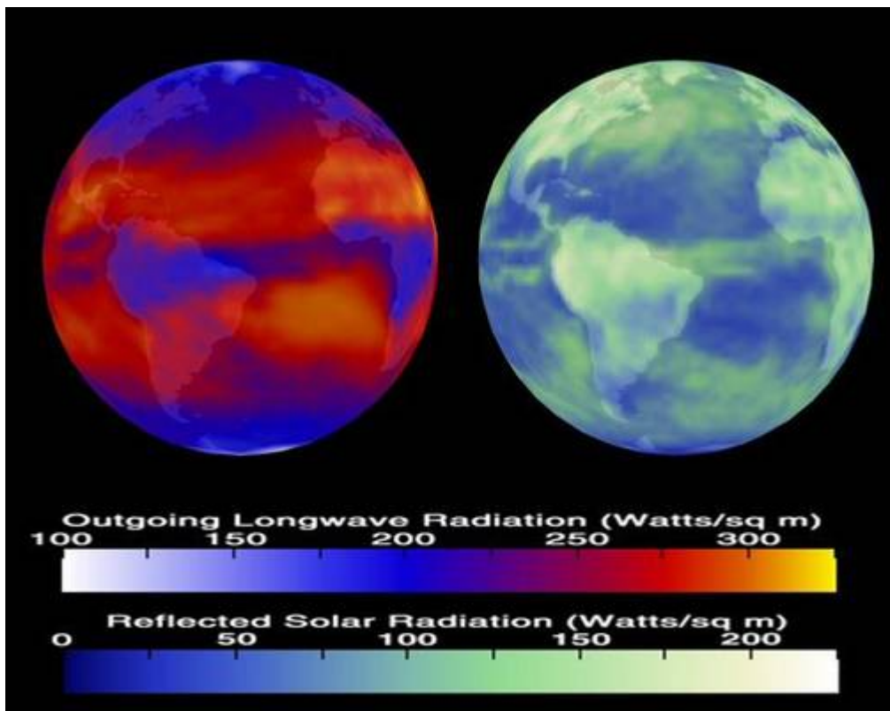
Abbildung 2: Terra/CERES-Ansicht der Welt bei der ausgestrahlten langwelligen Strahlung (links) und des reflektierten Sonnenlichtes (rechts). Bild: NASA.
