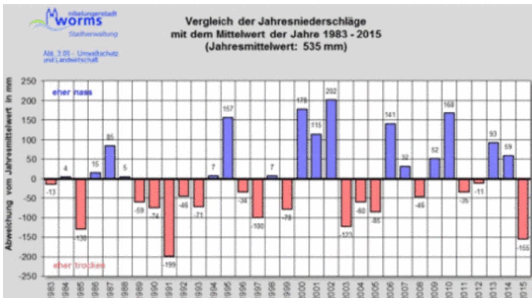
Bild 24 Niederschlag Stadt Worms von 1983 – 2015. Quelle: Stadt Worms 2016: Konzept zur Anpassung an den Klimawandel
