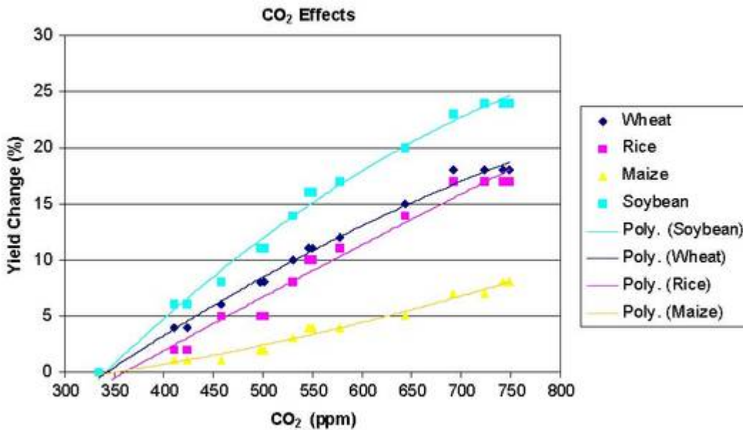
Abbildung 4: Zunahme des Ertrags von Nahrungspflanzen bei zunehmendem CO 2 aus der begutachteten Studie von Parry et al. [1].
