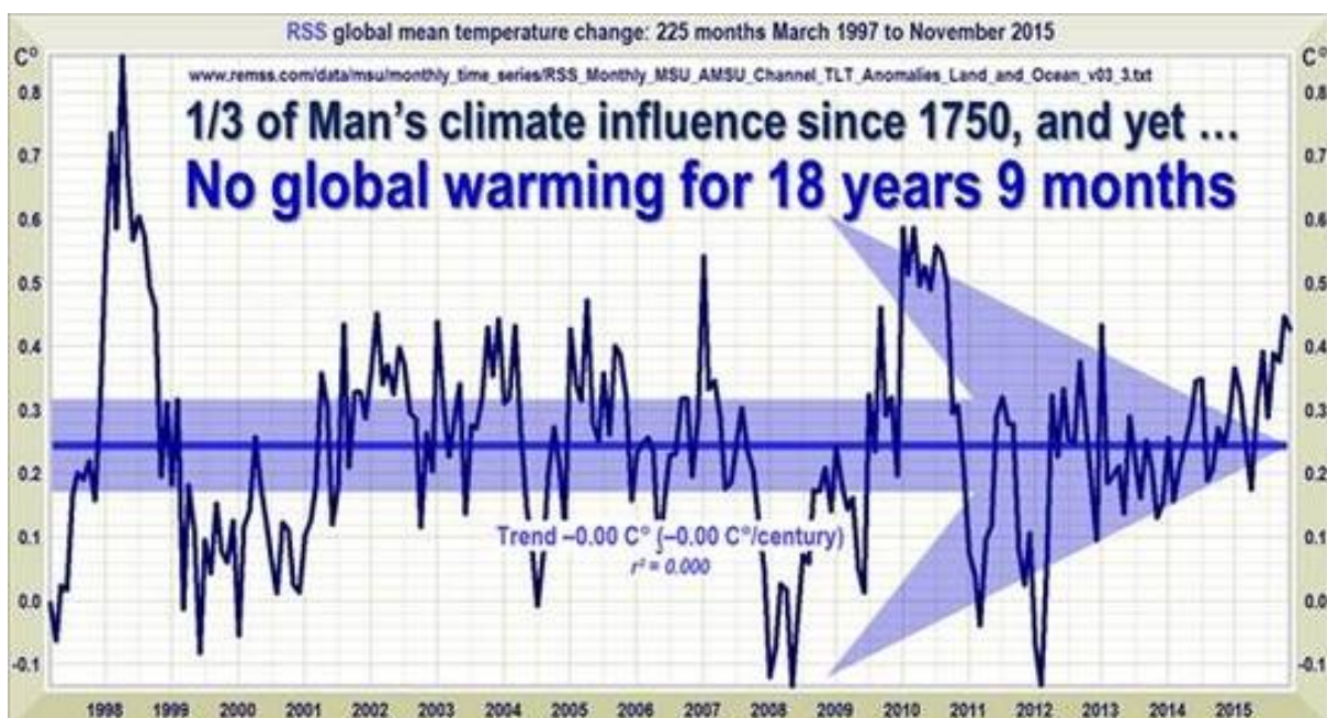
Abbildung 2: Temperaturverlauf und Trend nach RSS für die untere Troposphäre bis November 2015. Lesch sagt also die Unwahrheit, wenn er behauptet, dass die AfD Programm-Aussage nur den Trend bis Ende 2012 berücksichtigt hätte,
