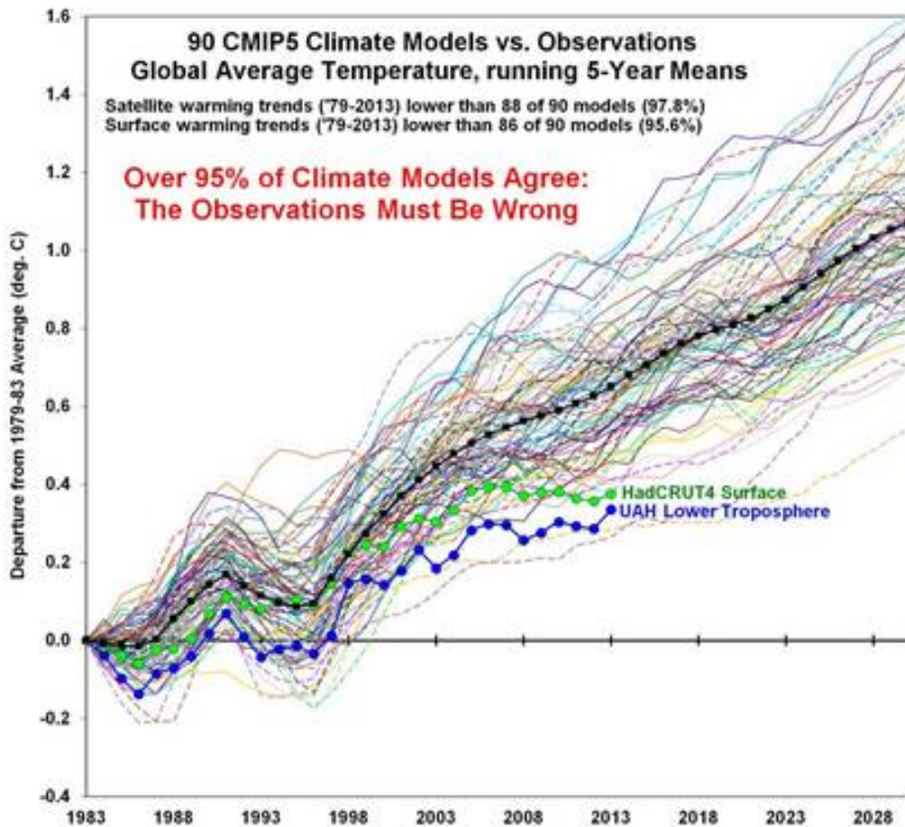
Abbildung 1: Modell Prognosen vs Beobachtungen (hier). 2 Modelle von 90 errechneten einen Verlauf der globalen Mitteltemperatur nahe den Beobachtungen durch Satelliten. Das liegt weit im Bereich des Zufalls. Nur 4 Modelle von 90 lagen unter den Trend der terrestrischen Messungen (Hadley CRU), die übrigens in Richtung Erwärmung zuvor „adjustiert“ wurden. 88 Modelle lagen zum überwiegenden Teil sehr massiv daneben. Gründe für die Abweichungen: unbekannt
