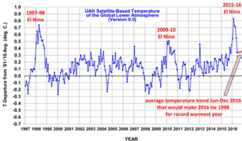
Abbildung 3: Temperaturverlauf und Trend nach UAH für die untere Troposphäre bis Juni 2016. Wichtig ist zu erkennen, dass die jeweils höchsten Spitzen 97/98; 2009/2010; und 2015/2016 von der gesamten Fachwelt dem El Niño Ereignissen zugeschrieben werden, von denen bisher noch niemand behauptet hat, sie würden durch die CO2 Emissionen ausgelöst. Derzeit liegen die Juni Temperaturen unter denen des El Nino Jahres von 1998, sollte sich das die Folgemonate jeweils fortsetzen, wird 2016 nicht als wärmstes Jahr in die Geschichte eingehen, meint jedenfalls jemand der es wissen muss: Roy Spencer (hier)
