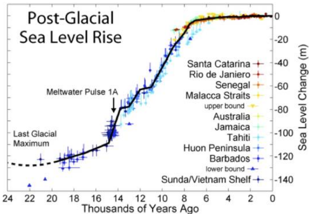
Abbildung 12: Anstieg des globalen Meeresspiegels seit dem Ende der
