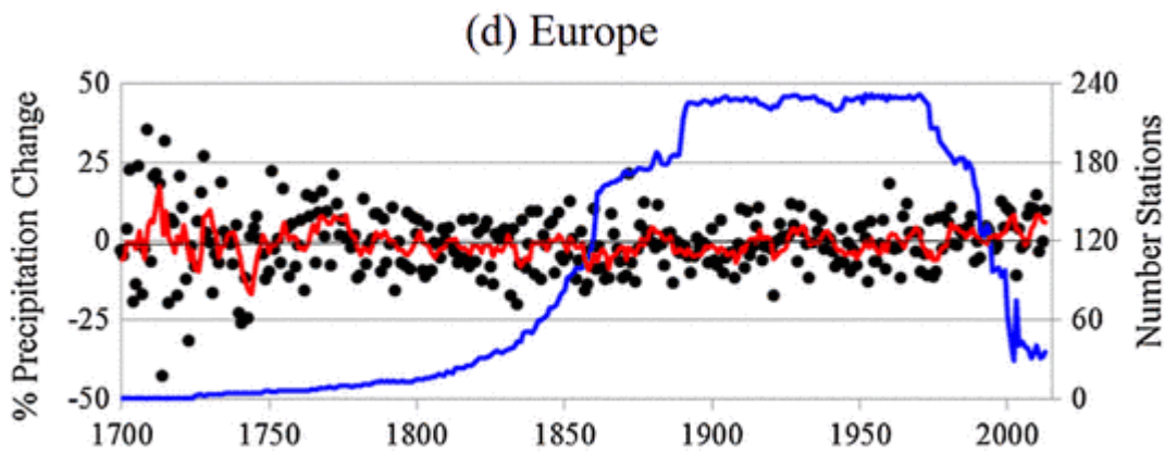
Bild 15 [6] Europa 1700 – 2013, relative Niederschlagsveränderung
