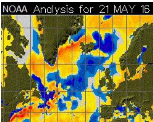
Abb. 8: Kaltwasserzone in Teilen des Nordatlantik (blau, negative Anomalien der Meeresoberflächentemperaturen von 0,5 bis etwa 3°C) als Vorzeichen einer baldigen Abkühlungsphase? Bildquelle: Amerikanischer Wetterdienst (NOAA)
