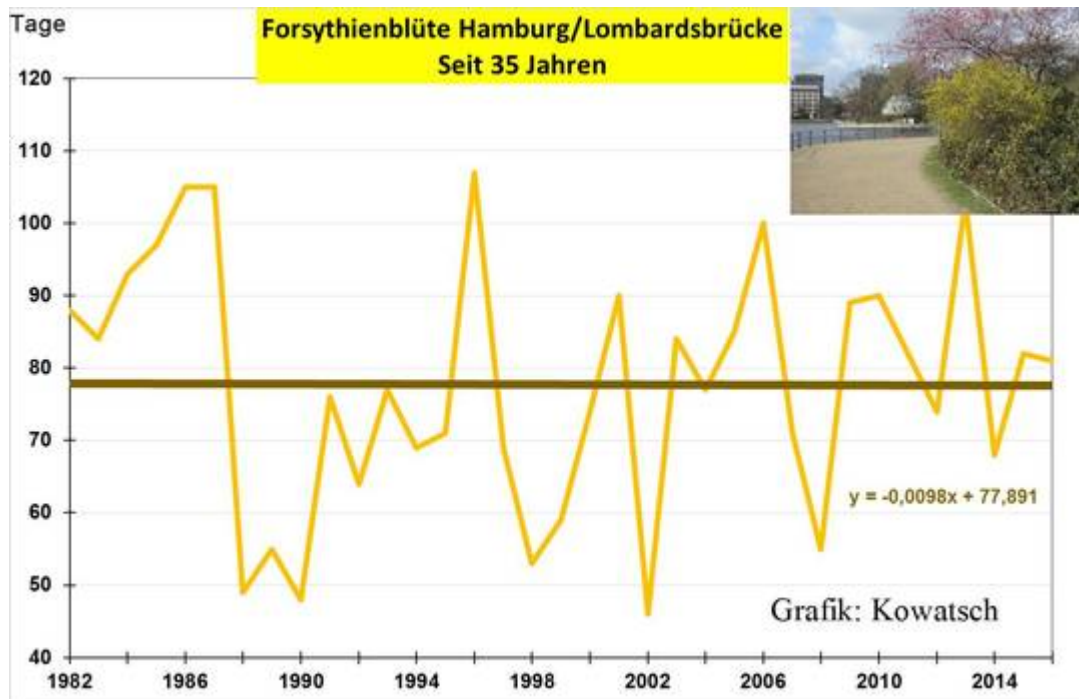
Abb. 13: Obwohl inmitten der großen Wärmeinsel Hamburg gelegen, stagniert der Eintritt der Forsythienblüte seit 35 Jahren. Ab 33 Jahren Betrachtung zeigt die Trendlinie bereits eine leichte Verspätung an. Für die Forsythienblüte sind die Temperaturen des Zeitraumes von Februar bis Anfang April ausschlaggebend.
