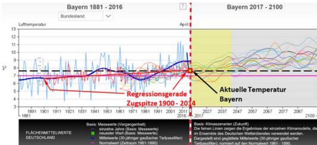
Bild 1 Temperaturverlauf Bayern. Vom Autor mit dem Verlauf der Zugspitze sowie Erklärungen und Hilfslinien ergänzt. Quelle: DWD Deutscher Klimaatlas Bayern
