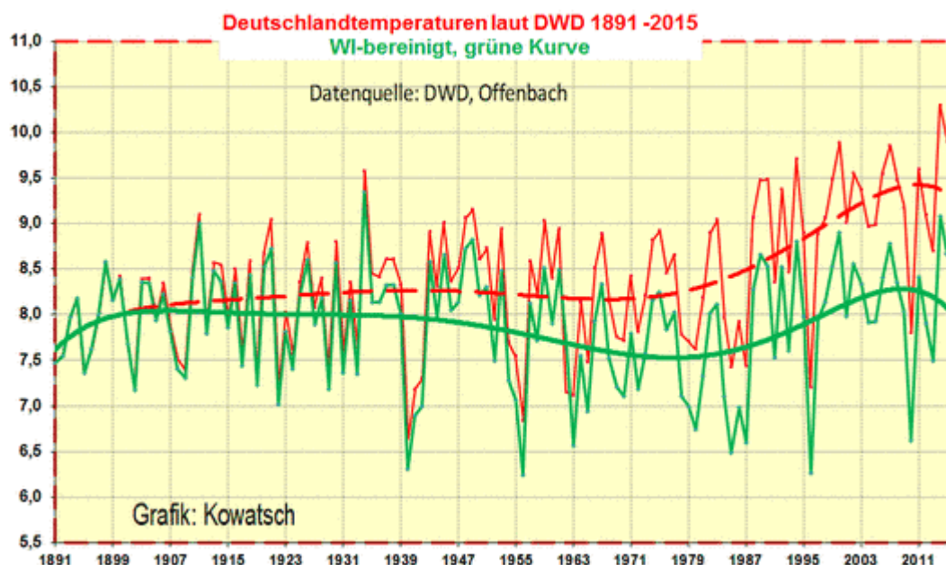
Grafik 1: Die von uns berechneten WI-bereinigten Deutschlandtemperaturen der letzten 125 Jahre
