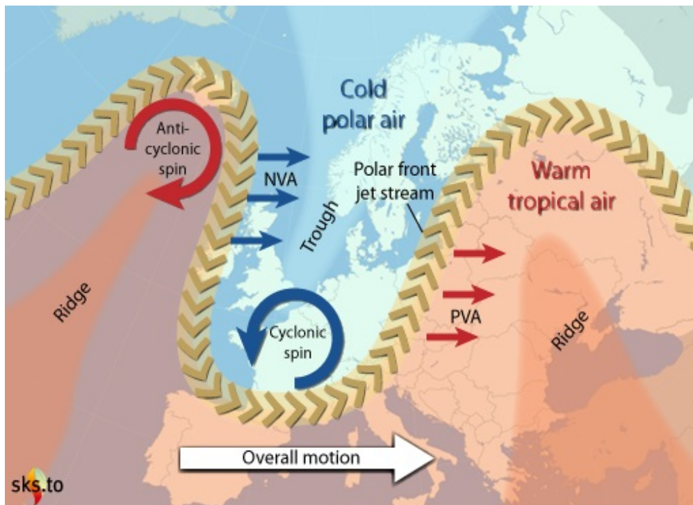
Abb.23b zeigt eine Momentaufnahme des PFJ und der Verteilung von Kalt und Warmluft, sowie die jeweiligen Windrichtungen, Quelle: John Mason.
