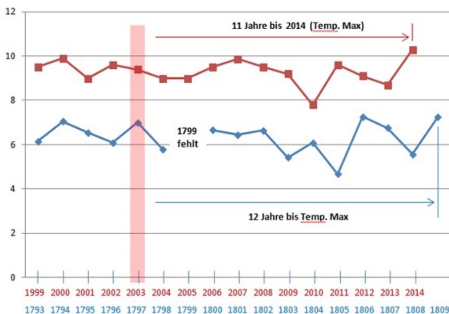
Abb.15 nach Daten des DWD zeigt den Temperaturgang der Temperaturreferenzstation HPB und die Deutschlandtemperaturen, jeweils
