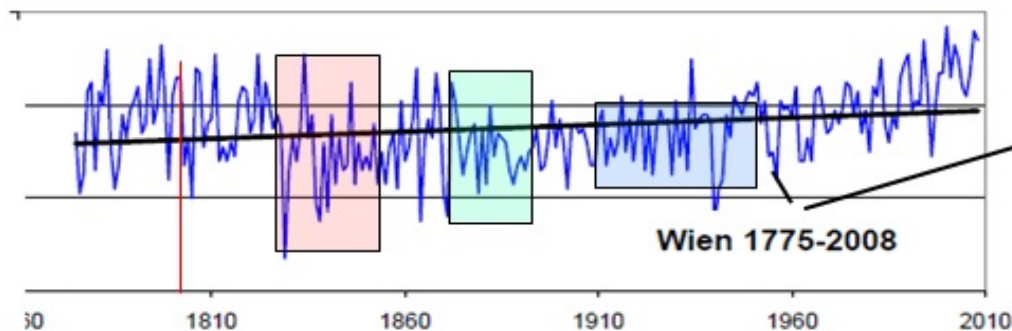
Abb.24: Zu sehen ist der Temperaturverlauf von Wien im Zeitraum von 1775 – 2008, Quelle: Prof. Ewert, EIKE. Die rote Linie gibt den Zeitpunkt des Maximums im Hauptsonnenzyklus an. Bis zu einem Zeitraum von 20 – 30 Jahren nach dem Hauptsonnenzyklus schwanken die Temperaturen am stärksten zwischen warm und kalt (rote Fläche). Bis zu dessen Minimum sind immer noch relativ hohe Temperaturschwankungen zu verzeichnen, jedoch auf insgesamt niedrigerem Niveau (grüne Fläche). Unmittelbar vor und nach dessen Minimum ist das Klimasystem sozusagen in seinem eingeschwungenen, kalten Zustand und die Ausschläge sind am geringsten.
