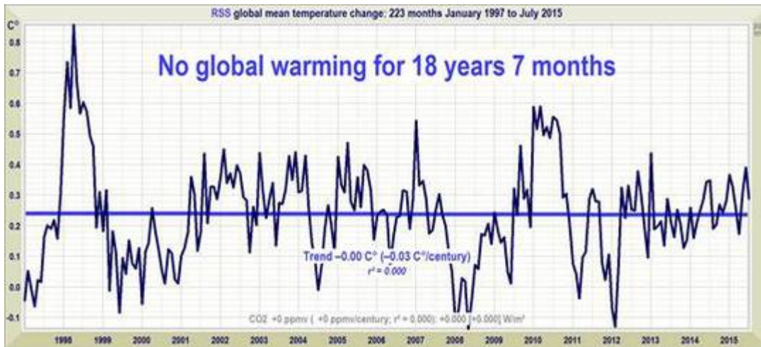
Abbildung 1: Die lineare Regression kleinster Quadrate des Trends der globalen monatlichen Temperaturanomale nach RSS zeigt keine globale Erwärmung seit 18 Jahren und 7 Monaten, also seit Januar 1997.
