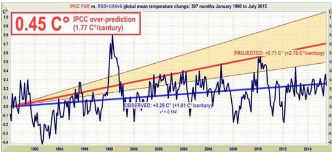
Abbildung 2: Echtzeit-Projektionen der Erwärmung mit einer Rate äquivalent zu 2,8 (1,9; 4,2) K pro Jahrhundert, erstellt mit „substantiellem Vertrauen“ des IPCC im Jahre 1990 für die 307 Monate von Januar 1990 bis Juli 2015 (orangefarbener Bereich und rote Trendlinie) im Vergleich zu gemessenen Anomalien (dunkelblau) und Trend (hellblau) mit einem Äquivalent von nur 1 K pro Jahrhundert, gemittelt aus den Satelliten-Datensätzen von RSS und UAH.
