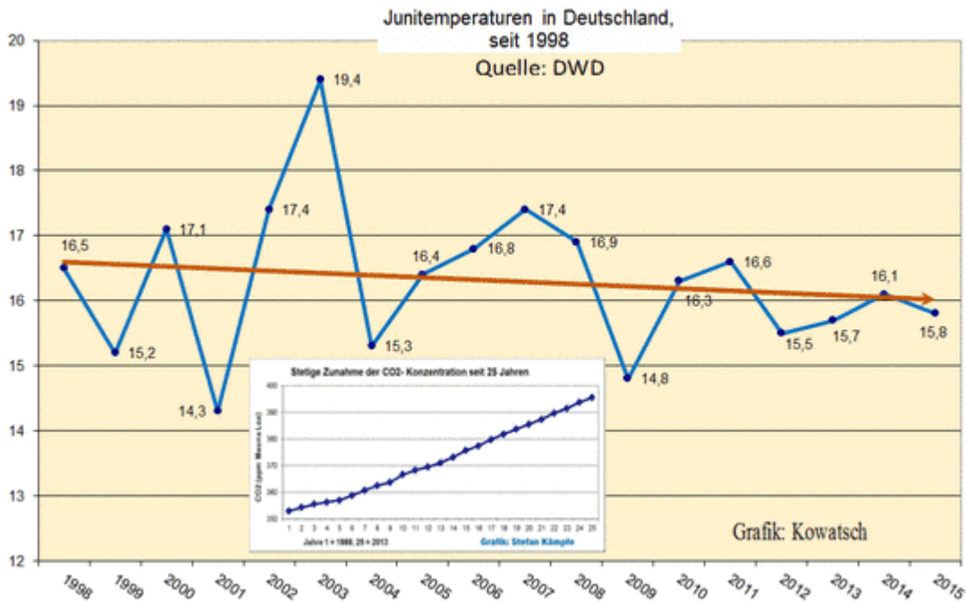
Abb. 13: Abkühlung im Juni. Auch der Juni 2015 ordnete sich entlang der fallenden Trendlinie ein. Der Juni wird kälter, der Juli wärmer und der August wieder kälter, also 2 zu 1 für die Kälte. Genau das zeigen auch die Sommertemperaturen seit 1998.
