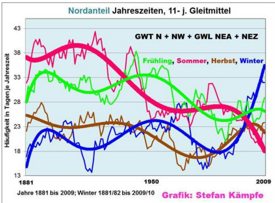
Abb. 10 und 11: Im Sommer nahm die Häufigkeit südlicher Lagen (obere Abb.) besonders zu, die der (normalerweise) viel sommertypischeren nördlichen Lagen hingegen ab (untere Abb.). Nur der Winter blieb ohne Zunahme südlicher Strömungen; dafür wurden in der kalten Jahreszeit nördliche Strömungen häufiger- eine wesentliche Ursache, warum sich der Winter in Deutschland während der vergangenen fast 30 Jahre leicht abkühlt.
