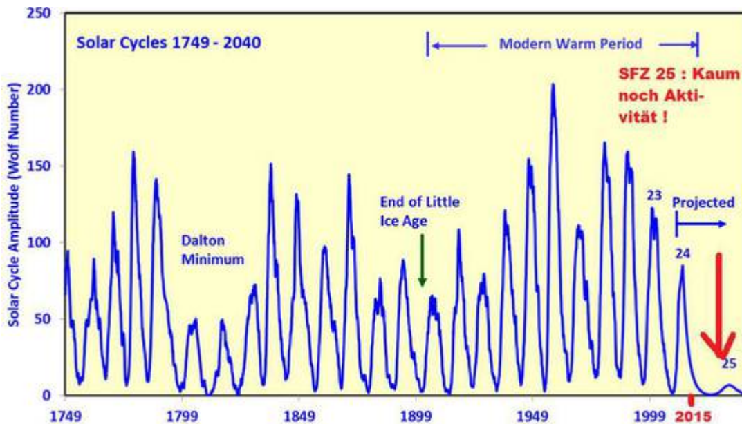
Abb. 4: Die Sonnenaktivität im Rhythmus des etwa 11jährigen SCHWABE-Zyklus. Man erkennt die besonders hohen Maxima ab der Mitte des 20. Jahrhunderts. Der letzte Zyklus Nr. 24 verlief deutlich schwächer, und der kommende Zyklus 25 (rechts am Bildrand, roter Pfeil) könnte extrem schwach verlaufen oder gänzlich ausfallen.
