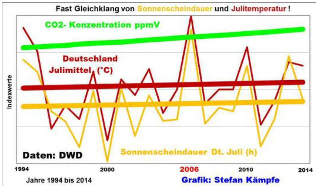
Abb. 2: Fast völliger Gleichklang von Juli- Temperaturen und Sonnenscheindauer. Der bislang heißeste Juli in Deutschland (2006) wies auch die meisten Sonnenstunden auf. Sehr sonnig waren auch die anderen warmen Juli- Monate 1994, 1995, 1999, 2001, 2010 und 2013. Der kälteste Juli seit 1994 (2000) war auch der sonnenscheinärmste; auch der zweitkälteste Juli (2011) verlief sehr trüb. Die stark steigenden CO 2 -Werte (oberste, grüne Linie) hatten offenbar keinen wesentlichen Einfluss auf die Juli- Temperaturen.
