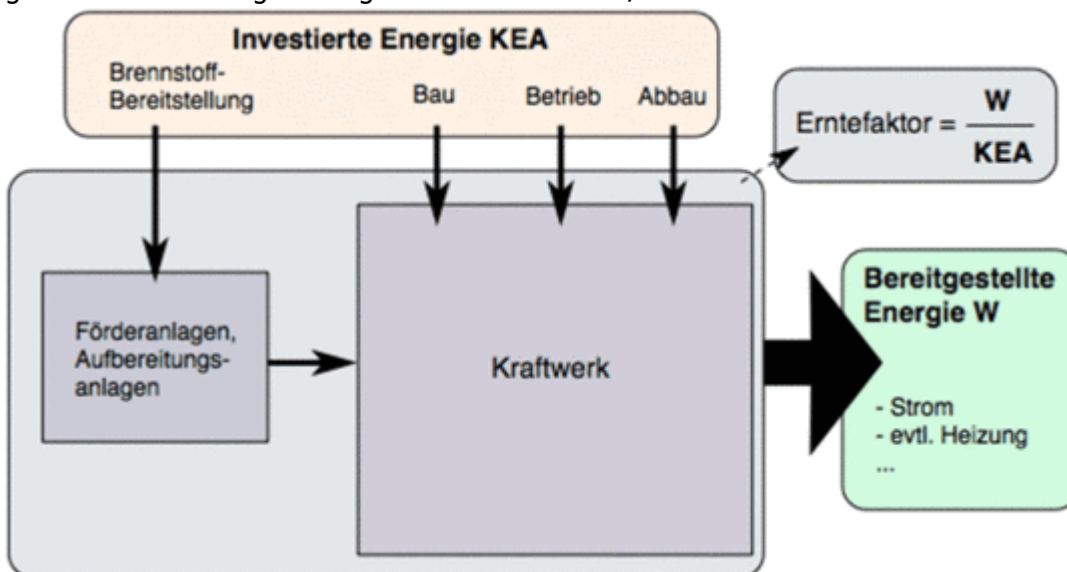
Bild 1. Der Erntefaktor eines Kraftwerks. Die Brennstoffbereitstellung (Förderung, Aufbereitung, usw.) findet normalerweise außerhalb des eigentlichen Kraftwerks statt, wird aber fairerweise zur investierten Energie hinzugerechnet (Grafik: [FEST])
