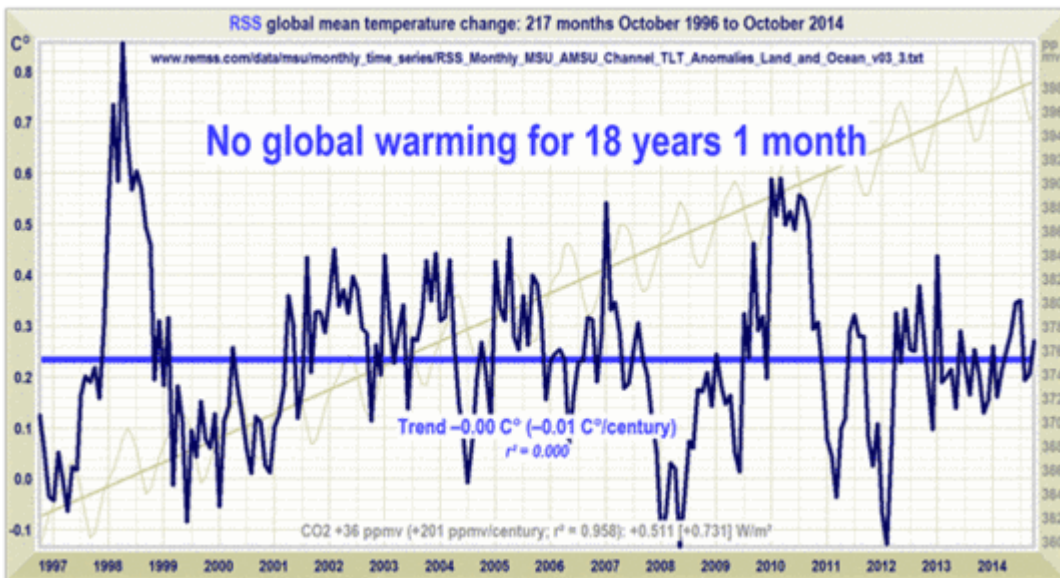
Abbildung 2: Die lineare Regression kleinster Quadrate des Trends im globalen RSS-Satelliten-Datensatz der monatlichen mittleren globalen Temperaturanomalien zeigt seit Oktober 1996, also seit 18 Jahren und 1 Monat, keinerlei Erwärmung. Die Stillstandsperiode von 18 Jahren und 1 Monat, also 217 Monate ist der am weitesten zurück reichende Zeitraum mit Satelliten-Temperaturmessungen und zeigt immer noch keinen von Null unterscheidbaren Trend.
