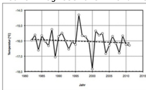
Abb.5 [14] Temperatur-Abkühlungs-Trend an der NEUMAYER-Station
