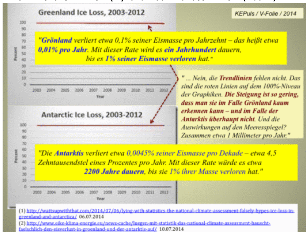
Abb.1 Trends der Eis-Massen [5]
