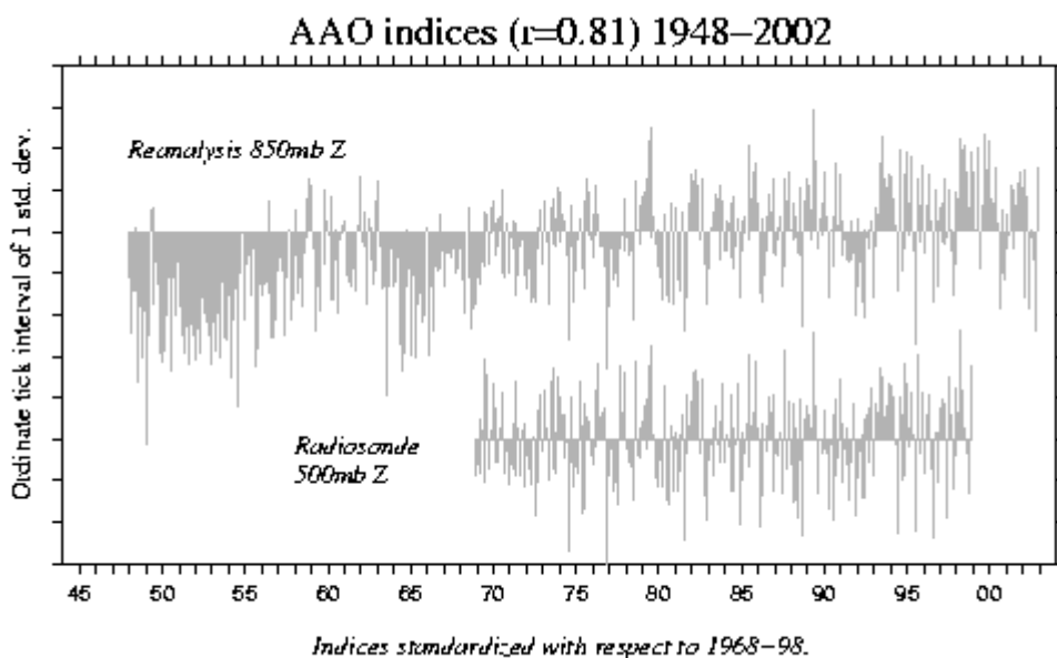
Abb.3 [10] Antarktische Oszillation
