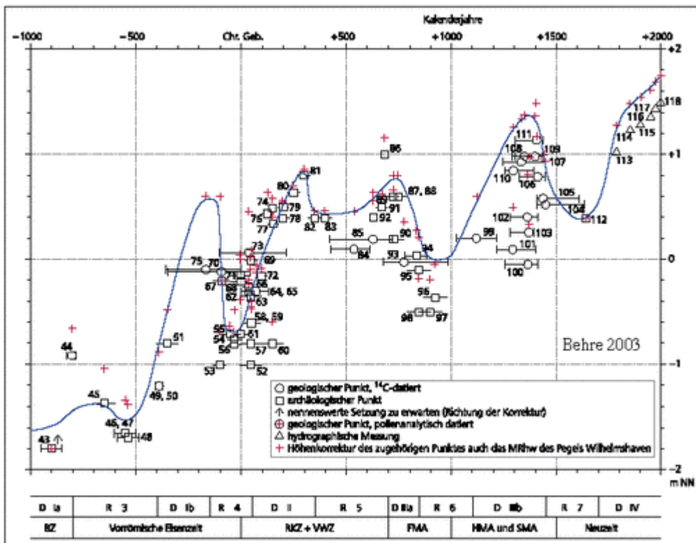
Abbildung 2 [1a (2003), S.35] Meeres-Anstieg für die südliche Nordsee der letzten 3.000
