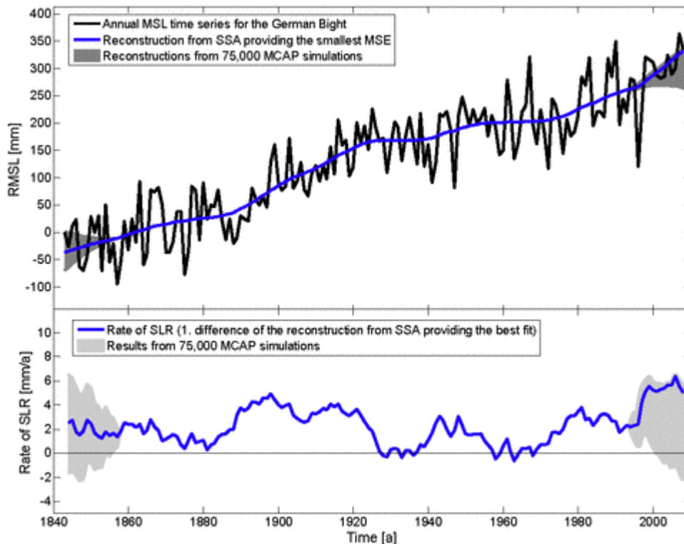
Abbildung 4 a+b [7a] Trends von 15 Küsten-Pegeln Deutsche
