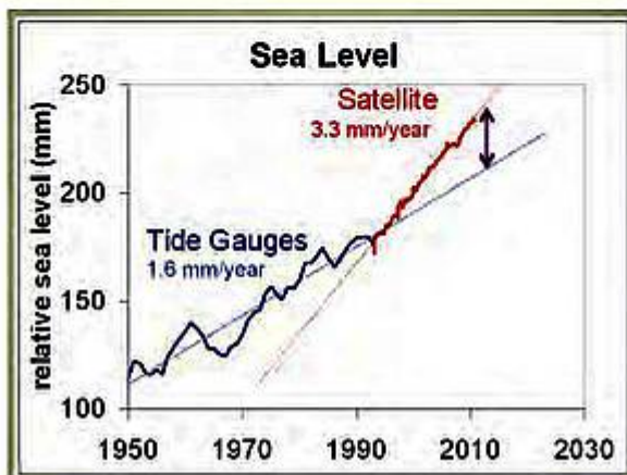
Abbildung 11 a+b: Gegenüberstellung der Pegel- und Sat-
