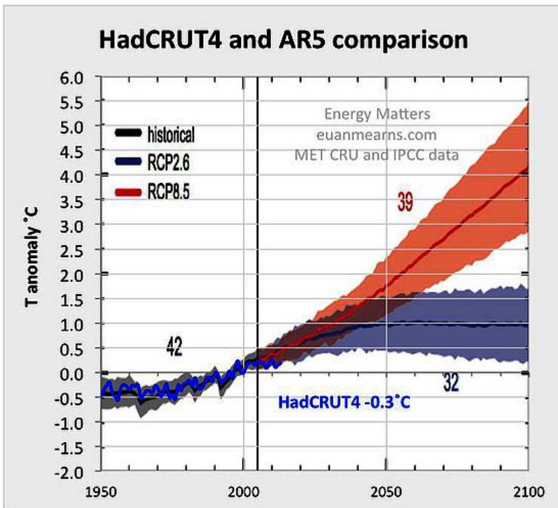
Abbildung 11: Vergleich der Realität mit Modellszenarien aus dem AR 5. Mit Modellbeginn im Jahre 2005 haben wir nur 8 Jahre, um die Modelle mit der Realität zu vergleichen. Dieses Mal muss ich von HadCRUT4 0,3°C abziehen, um Übereinstimmung mit den Modellen zu erreichen. Vor 2005 bilden die Modelle vermeintlich die Realität seit 1950 ab. Vor 1950 wird uns eine Ansicht verwehrt, wie die Modelle damit aussahen. Nach 2005 ist klar, dass die Realität entlang der unteren Grenze der Bandbreite der beiden Unsicherheitsbereiche verläuft, die geplottet sind. Dies ist eine Beobachtung, die auch viele andere gemacht haben (z. B. 1).
