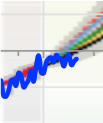
Abbildung 6: Die einzelne vertikale Gitternetzlinie ist das Jahr 2000. Die blaue Linie zeigt HadCRUT4 (Realität). Sie bewegt sich waagrecht, während alle Modelle einen Aufwärtstrend zeigen.
