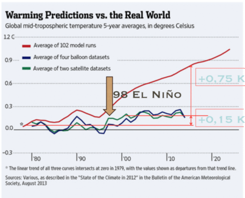
Abbildung 1: Vergleich der Entwicklung der mittleren Globaltemperatur in der Realität (Ballons & Satellitenmessungen) mit der CO 2 basierten Prognose (Szenarien) von 102 Klimamodellen bis 2025. Der Unterschied ist mit 0,6 K zu wenig mehr als deutlich
