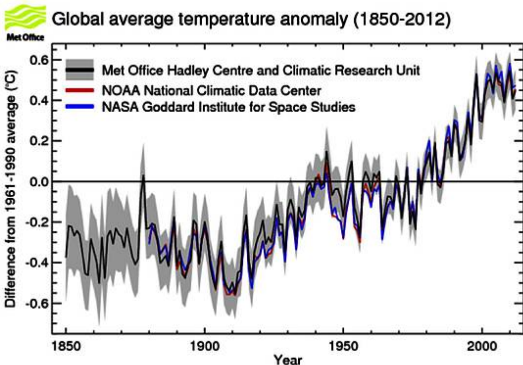
Abbildung 1: Anomalie der globalen Mitteltemperatur Quelle UK Metoffice
