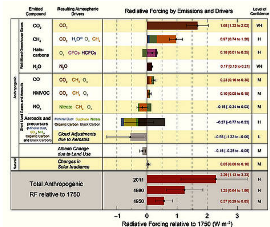
Abbildung 2: Art, Anzahl und Einfluss der Forcings lt. IPCC AR5 (Quelle Fig SPM 5 IPCC WG1 SPM)
