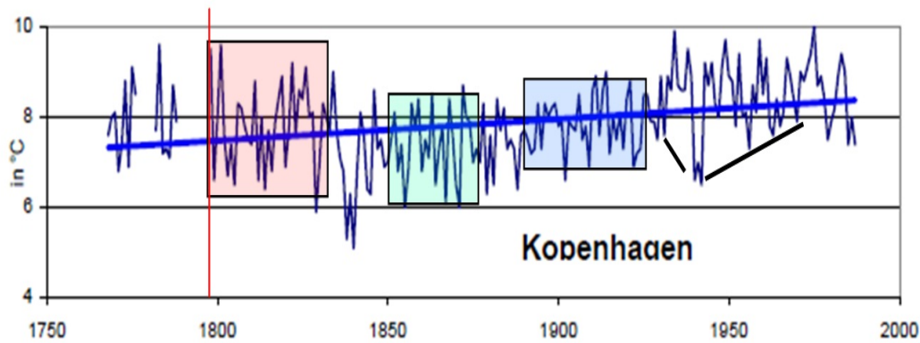
Abb. 15, Quelle: Prof. Ewert, EIKE, zeigt den Temperaturgang von Kopenhagen. Die rote Linie gibt den Zeitpunkt des Maximums im Hauptsonnenzyklus an. Bis zu einem Zeitraum von 20 – 30 Jahren nach dem Hauptsonnenzyklus schwanken die Temperaturen am stärksten zwischen warm und kalt (rote Fläche). Bis zu dessen Minimum sind immer noch relativ hohe Temperaturausschläge zu verzeichnen, jedoch auf insgesamt niedrigerem Niveau (grüne Fläche). Unmittelbar vor und nach dessen Minimum ist das Klimasystem sozusagen in seinem eingeschwungenen, kalten Zustand und die Ausschläge sind am geringsten. Vor einem Temperaturanstieg fallen die Temperaturen auf ein relatives Minimum und steigen dann kontinuierlich an (schwarze Linien).
