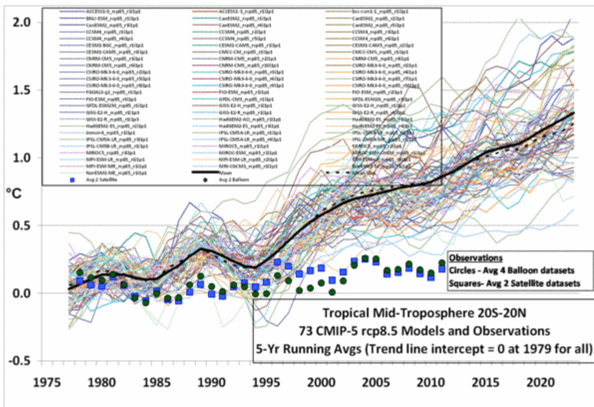
Abbildung 1: Prognosen der IPCC-Klimamodelle (dünne farbig Linien)
