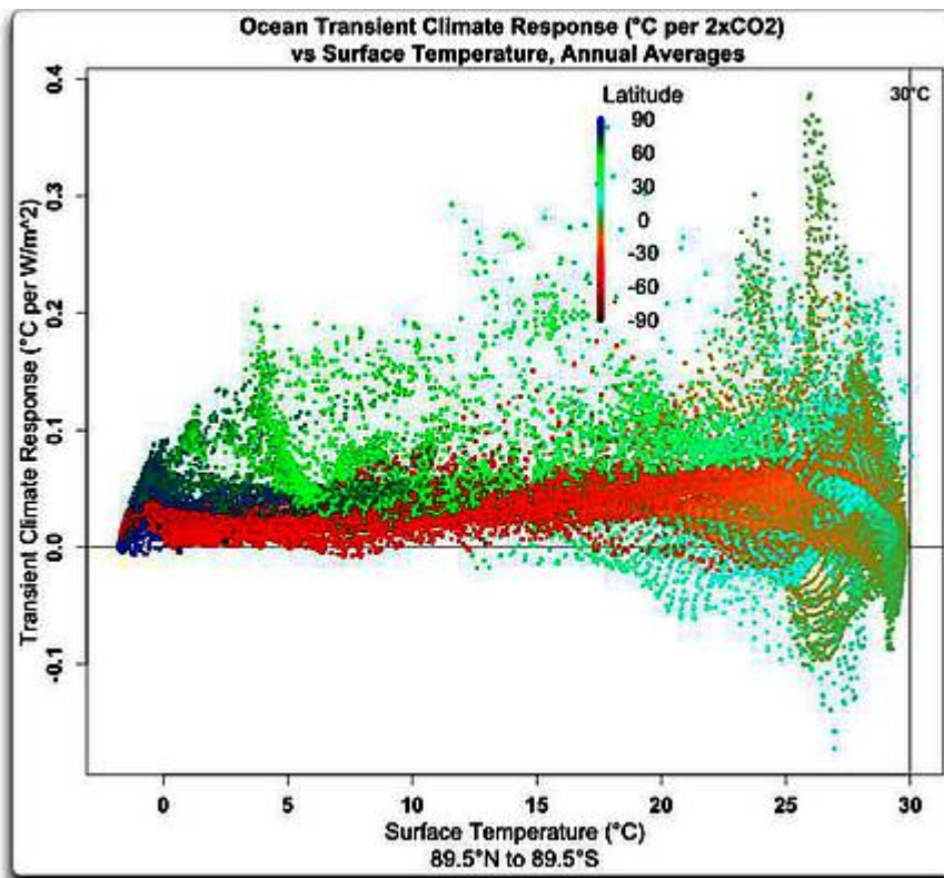
Abbildung 6: Wie in Abbildung 5, jedoch nur für den Ozean. Man beachte, dass sich die Skalierung von Abbildung 5 unterscheidet.
