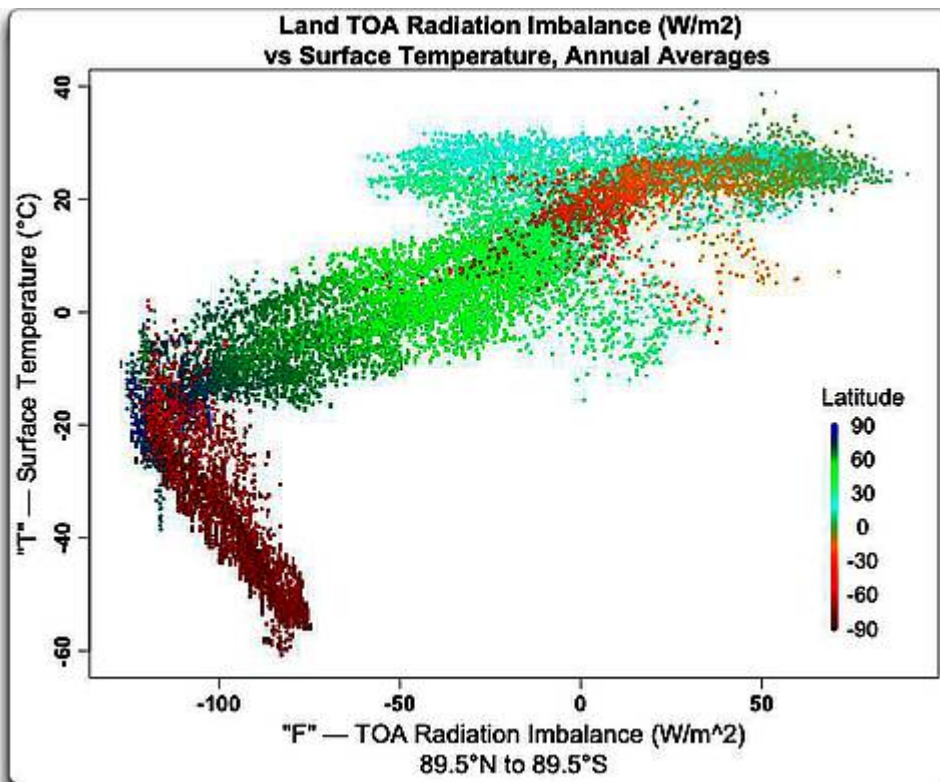
Abbildung 1: Festland allein, Antrieb F (Strahlungs-Ungleichgewicht an der TOA) und Temperatur T auf einem Gitternetz 1^\circ mal 1^\circ . Man beachte, dass zwischen 50^\circ\text{S} und 65^\circ\text{S} kaum Festland vorhanden ist. Der Gesamtantrieb an der TOA wird berechnet als einfallende Sonnenstrahlung minus langwellige Ausstrahlung.
