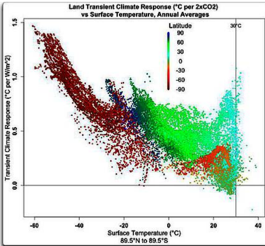
Abbildung 5: Transient Climate Response im Vergleich zur mittleren jährlichen Temperatur, nur Festland. Man beachte, dass TCR nur selten unter Null sinkt. Die größte Reaktion gibt es in der Antarktis (dunkelrot).
