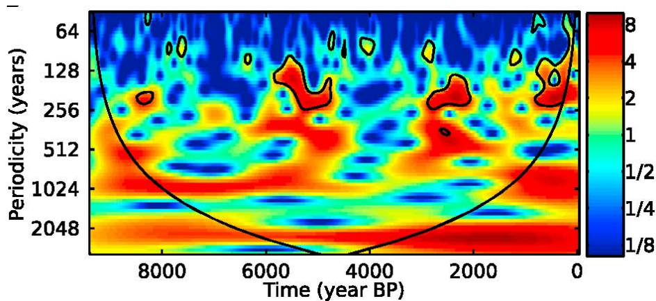
Bild 2: Waveletspektrum, die rechte Skala gibt die Stärke der Periodizität (in log2) an. Die schwarze Linie ist der "cone of influence", außerhalb von ihm werden die Ergebnisse allmählich unsicher. Der im Text erwähnte de Vries Zyklus, der in den letzten 1000 Jahre zu den stärksten Periodizitäten gehört, ist deutlich erkennbar.
