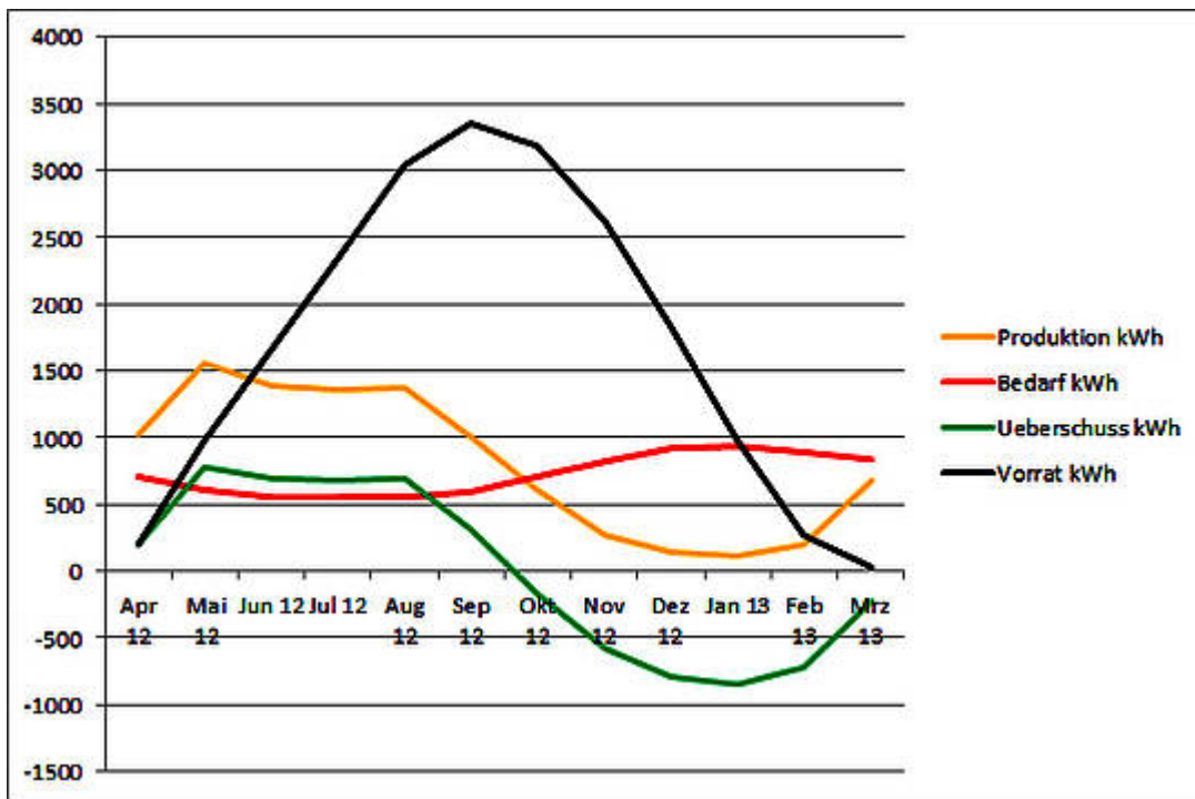
Bild 5. Simulation von Solaranlage und Batterien im Saisonspeicherbetrieb mit für Deutschland zwischen April 2012 und März 2013 ermittelten Solardaten
