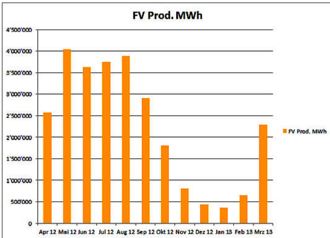
Bild 1: Solarstromproduktion in Deutschland im Zeitraum von April 2012 bis März 2013 in MWh (Datenquelle: EEX)
