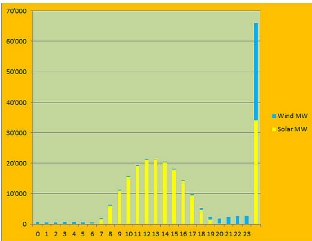
Bild 3. Erzeugung von Strom aus Wind- und Sonnenenergie in Deutschland am 22.8.2013. Teilweise sind es nur rund 600 MW, das reicht noch nicht einmal für den Standby-Betrieb der Nation. Ganz rechts die installierten Gesamtkapazitäten (Datenquelle: transparency.eex.com)
