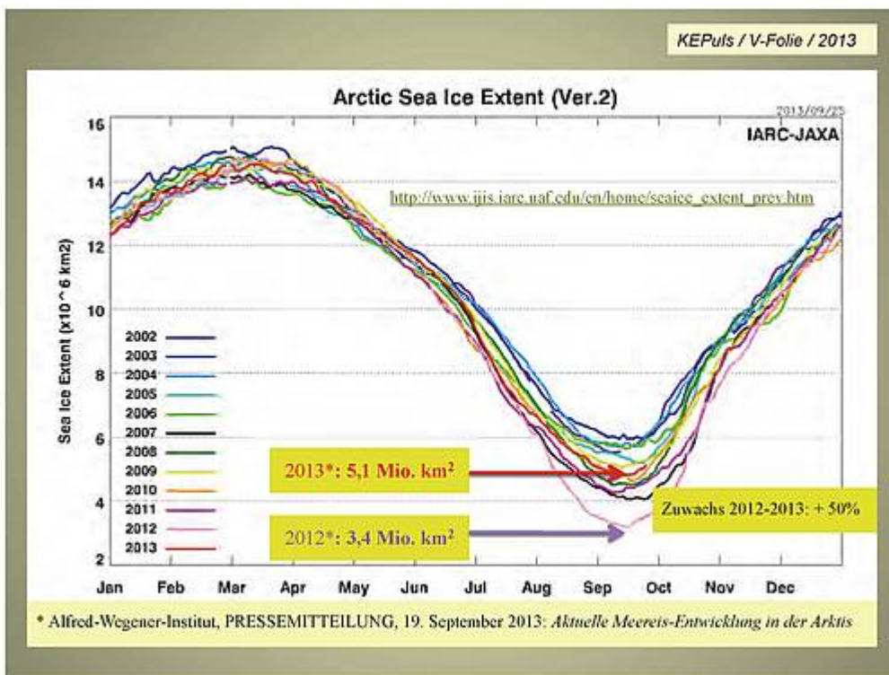
Abbildung 1 : Arktische Eisfläche 2002-2013 [6] Pfeile und Textfelder ergänzt
