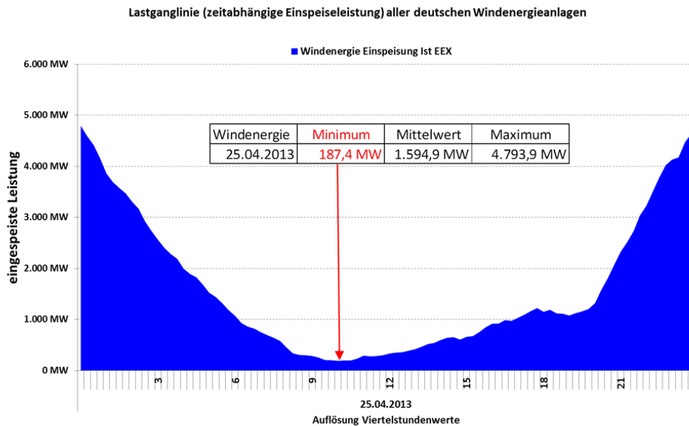
Abbildung 2: Gesamt-Windeinspeisung für den 25.4.13
