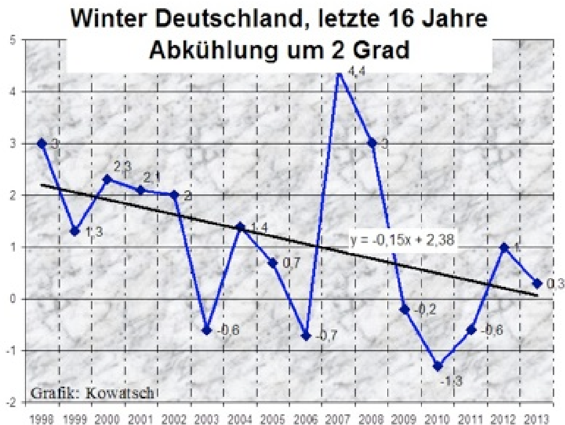
Abbildung 1[1] Winter-Temperaturen 1998-2013 (Dez.-Feb.) in Deutschland (Graphik J.KOWATSCH, Daten DWD)
