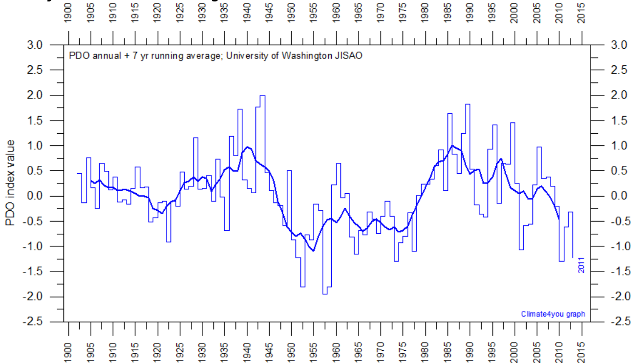
Abbildung 3 (Quelle: http://www.climate4you.com/ )
