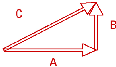
Abb. 4: Vektoren
